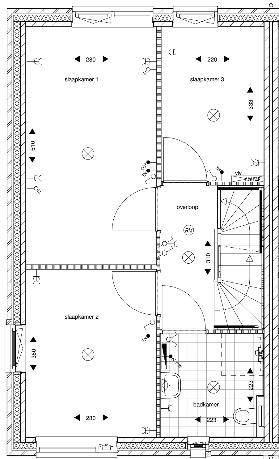
eerste verdieping
