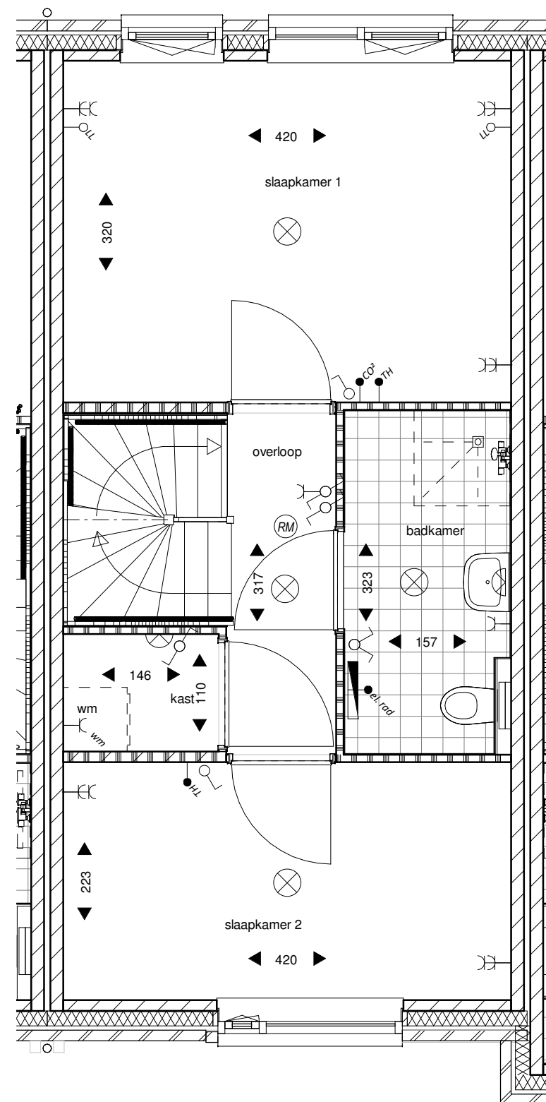
eerste verdieping
