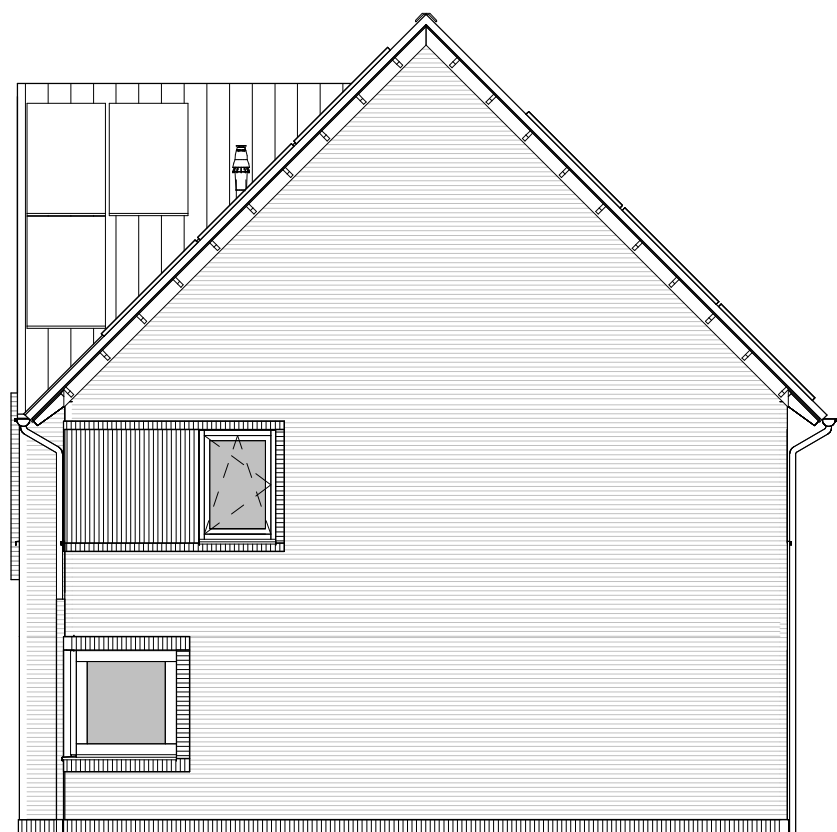
rechtergevel
