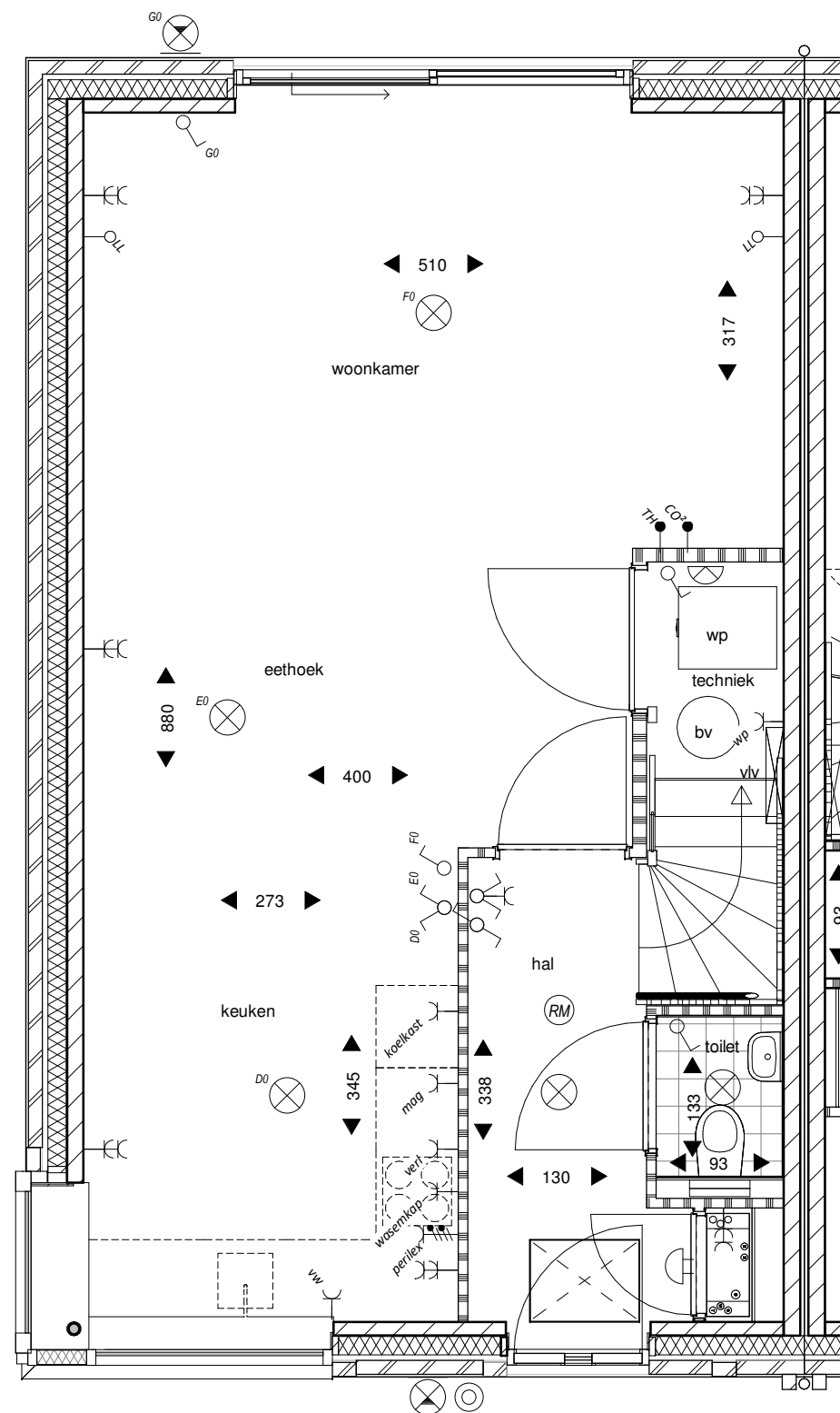
begane grond
