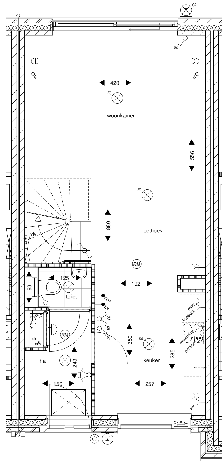
begane grond
