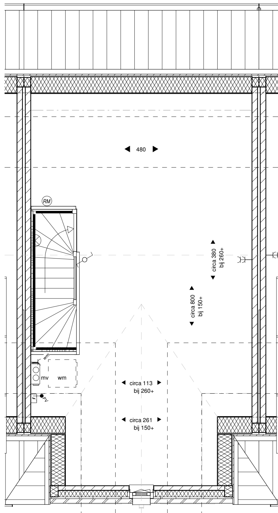
tweede verdieping
