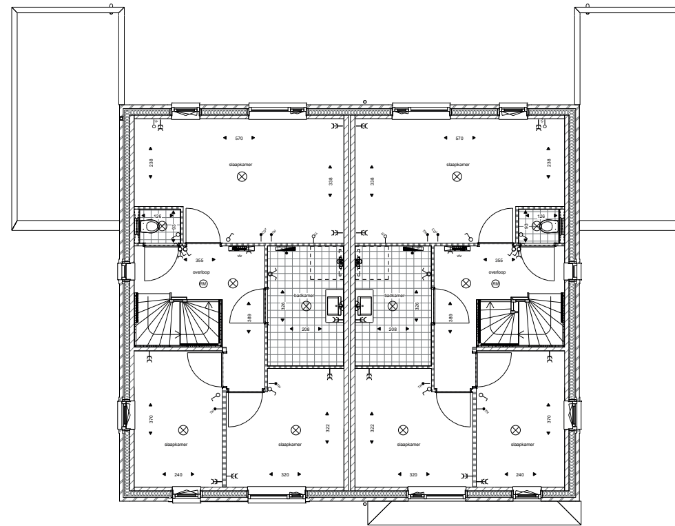
Eerste verdieping
