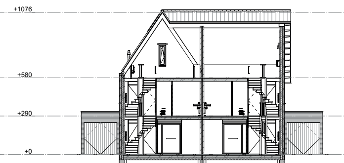
Doorsnede B
