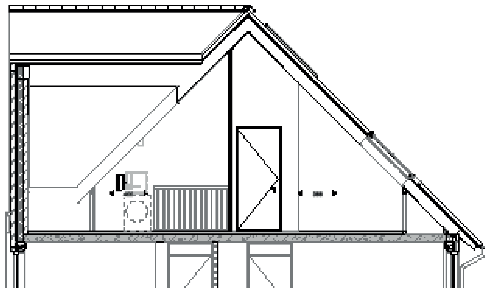
Doorsnede
