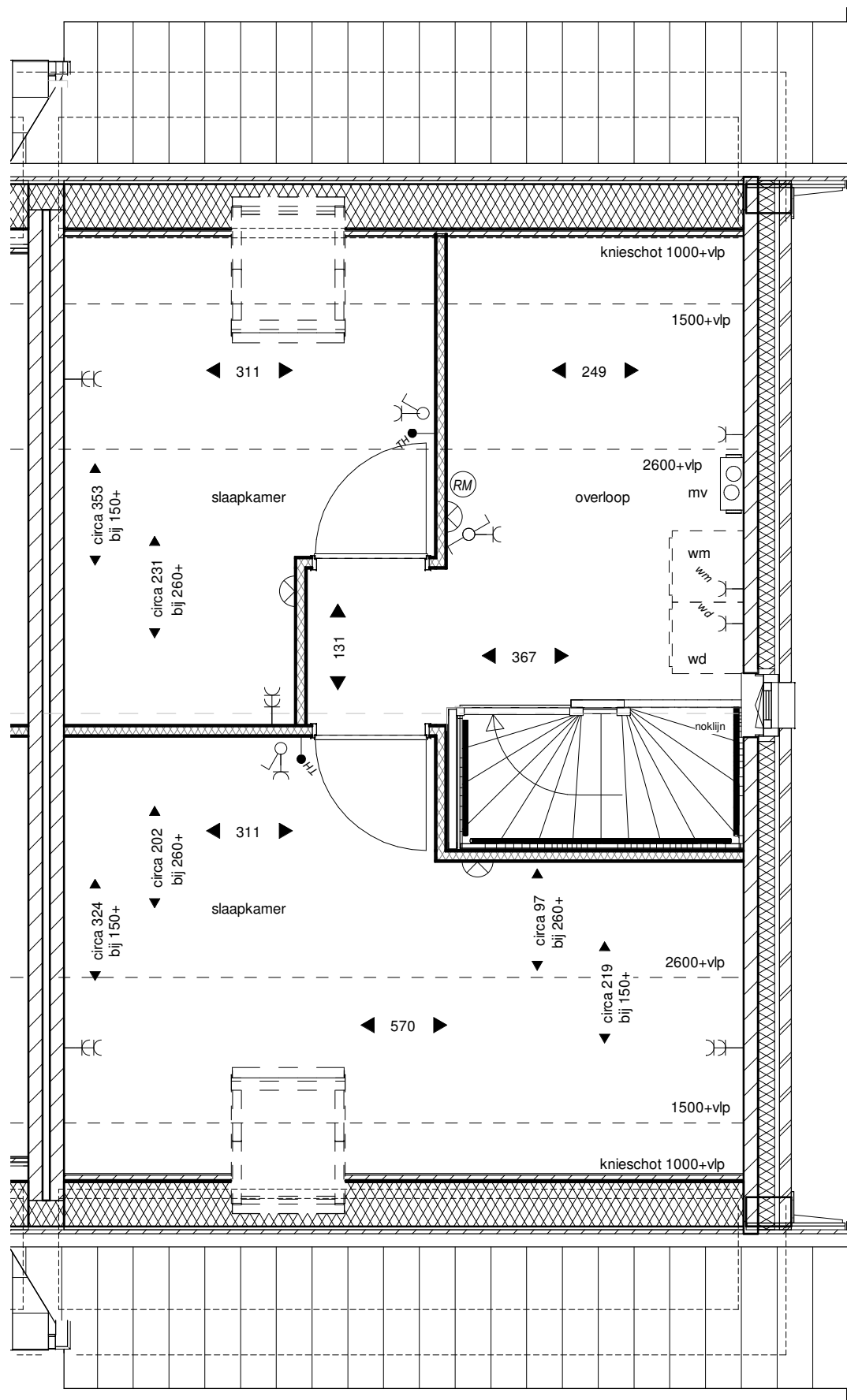
Tweede verdieping
