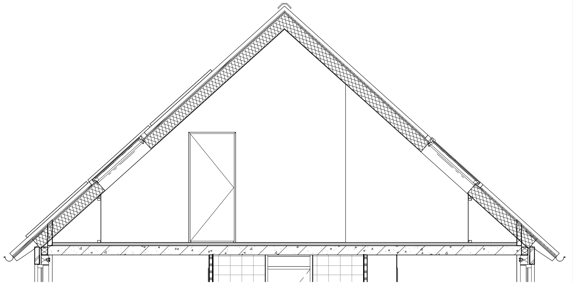
Doorsnede
