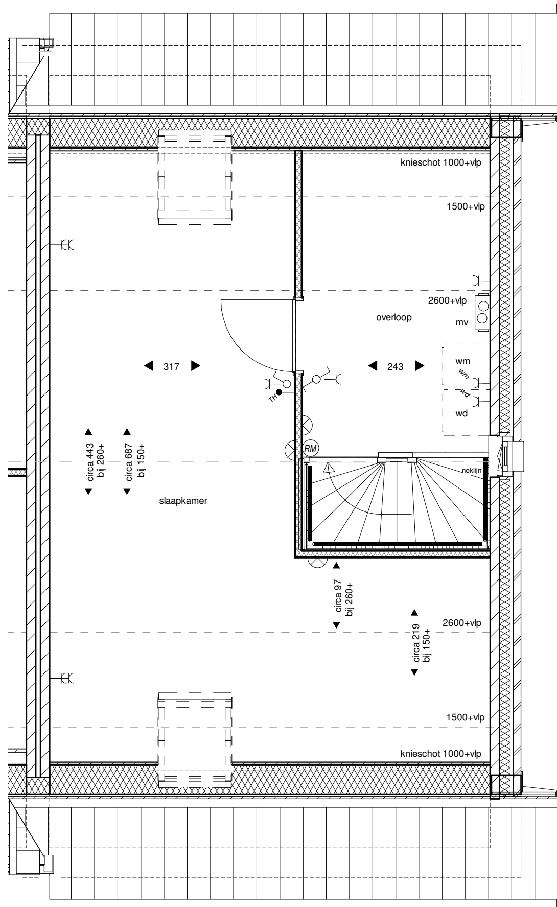
Tweede verdieping
