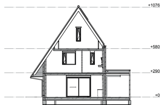
Doorsnede A
