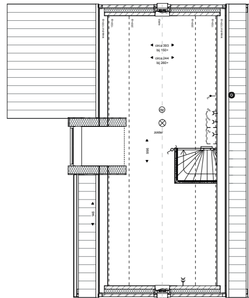
Tweede verdieping bouwnr 36
