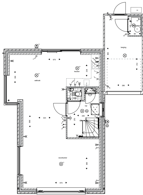
Begane grond bouwnr 36
