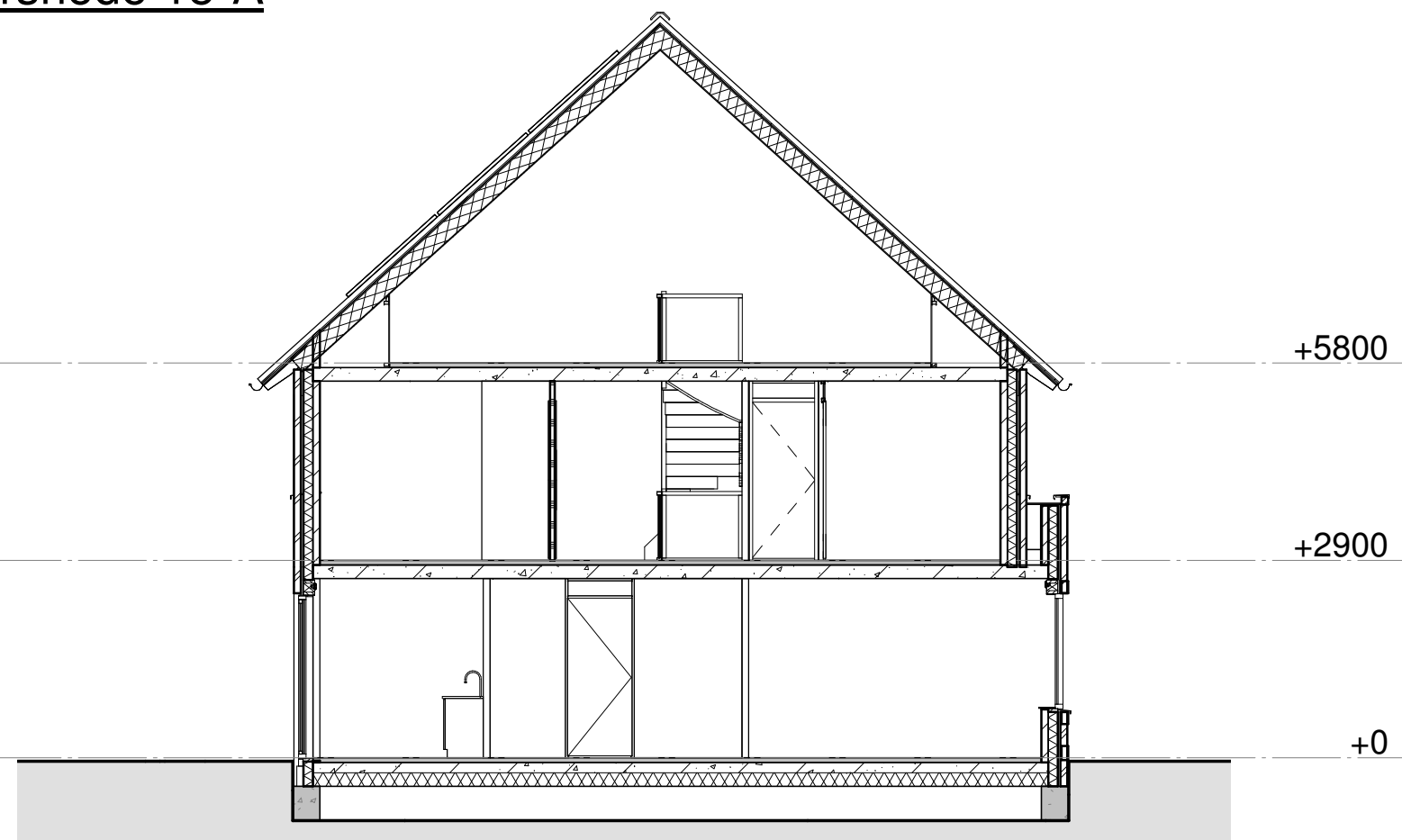
Doorsnede 15-A
