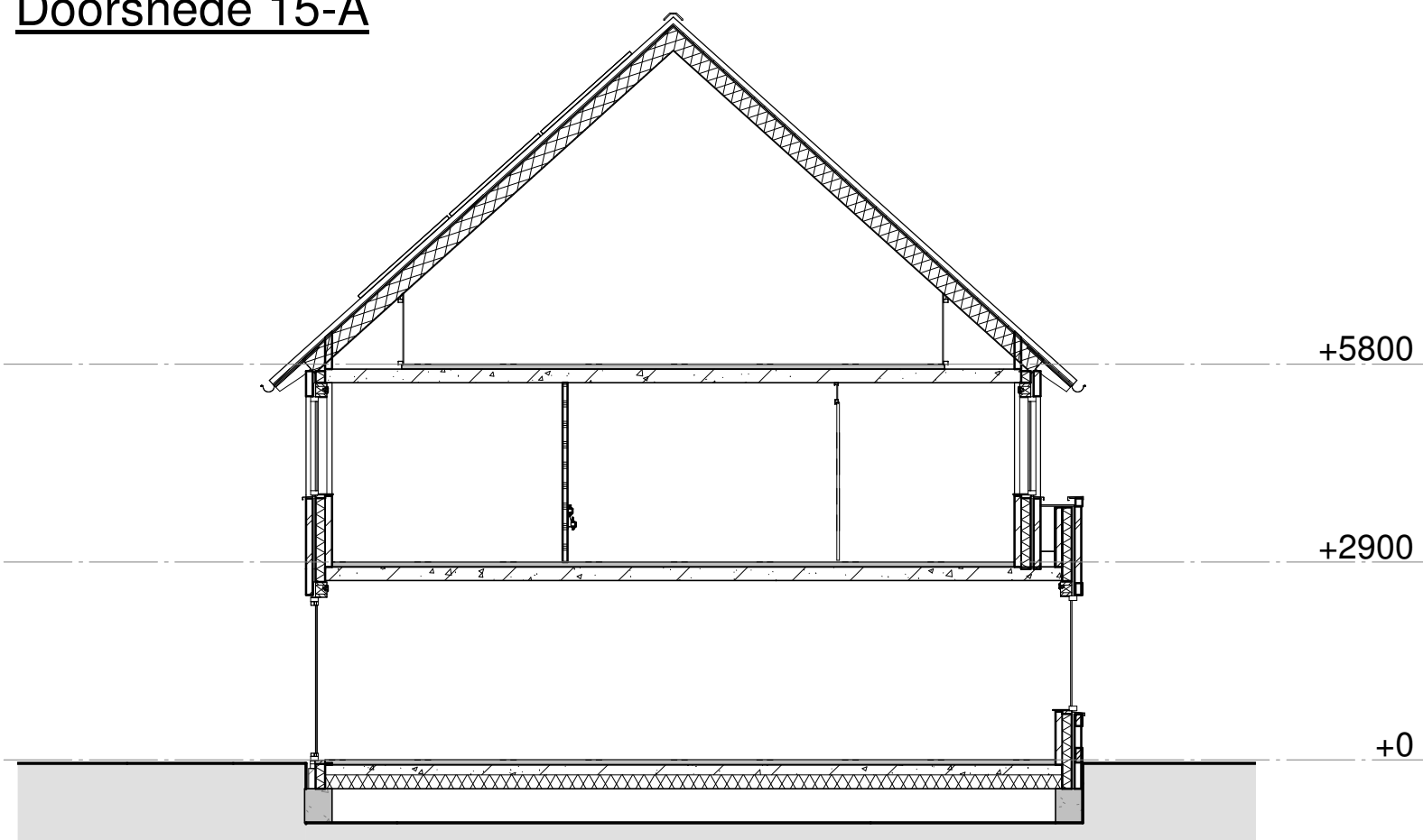
Doorsnede 15-B
