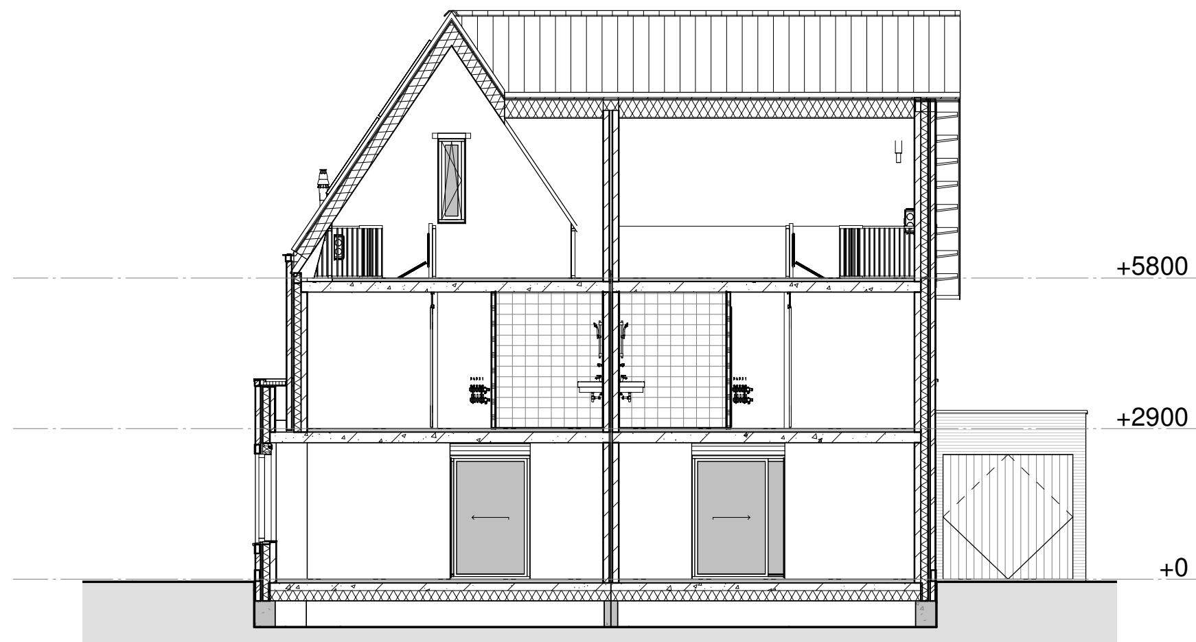
Doorsnede 15-A
