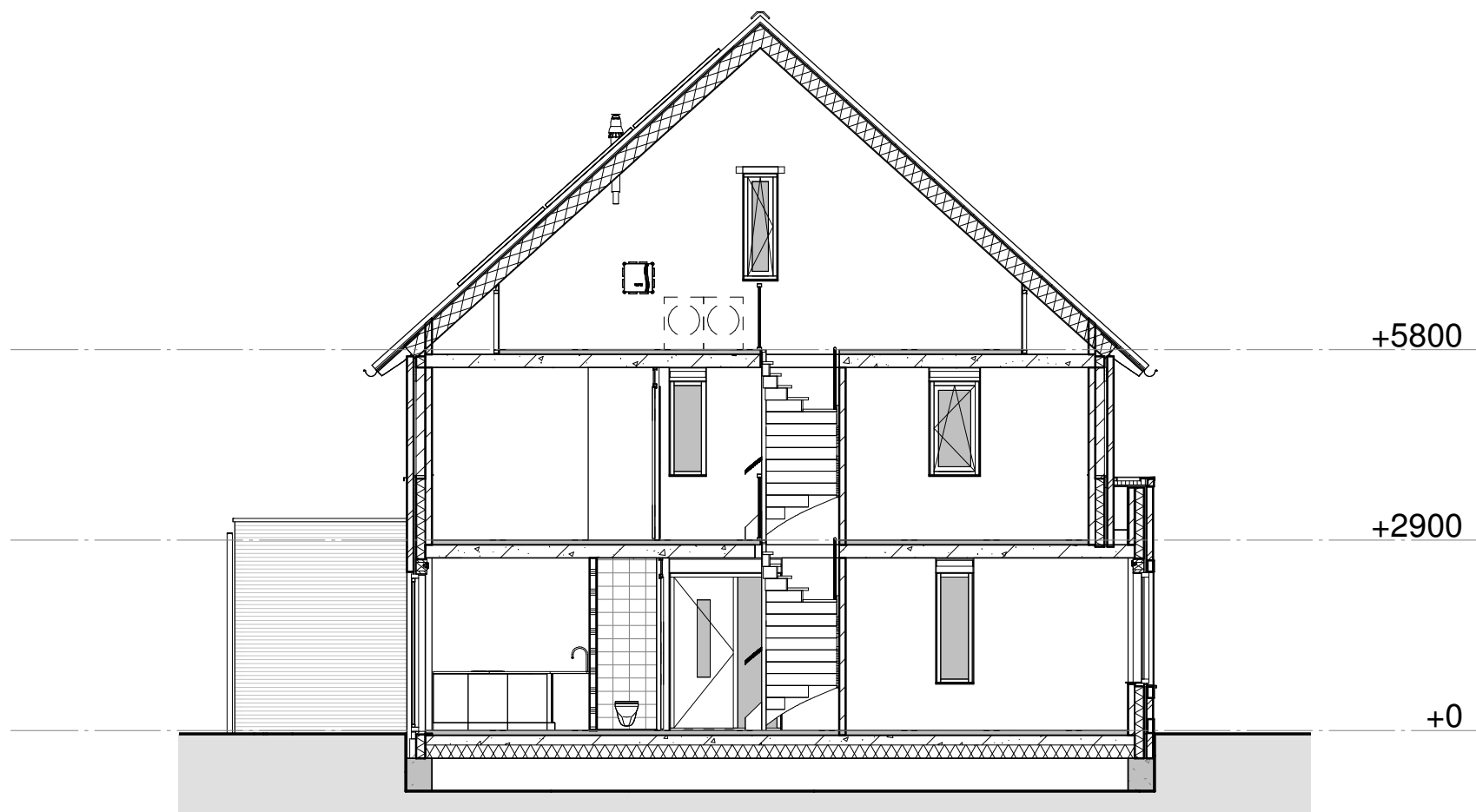
Doorsnede 15-A
