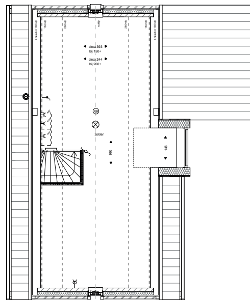
Tweede verdieping
