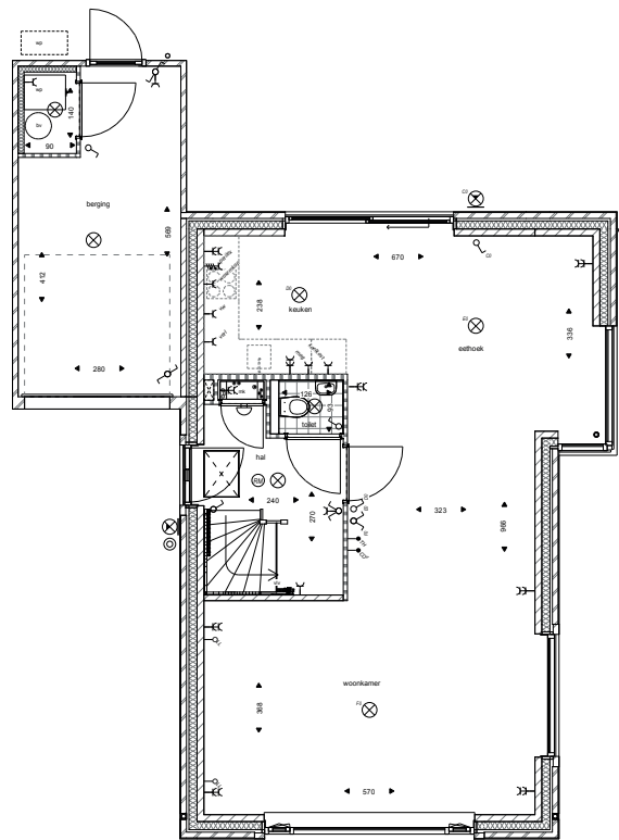
Begane grond
