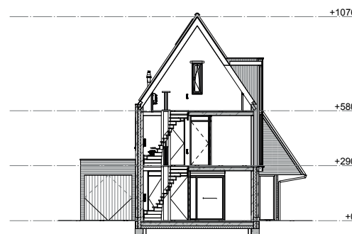
Doorsnede A
