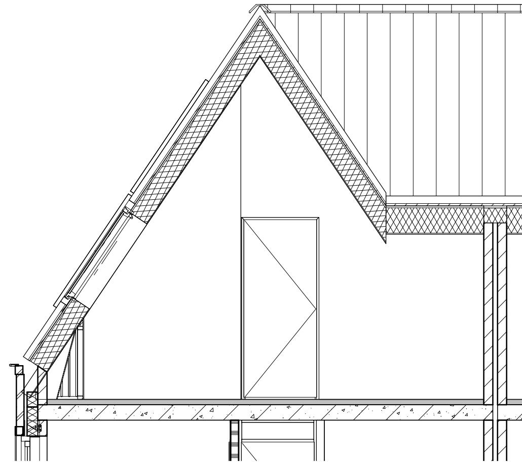
Doorsnede
