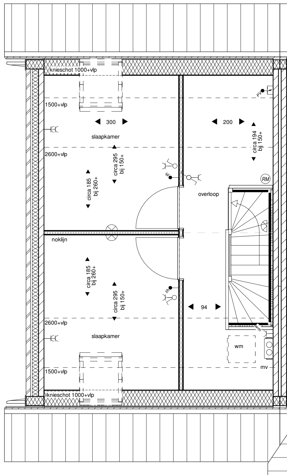
Tweede verdieping
