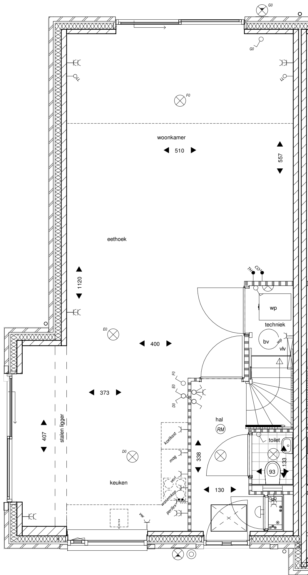
Begane grond
