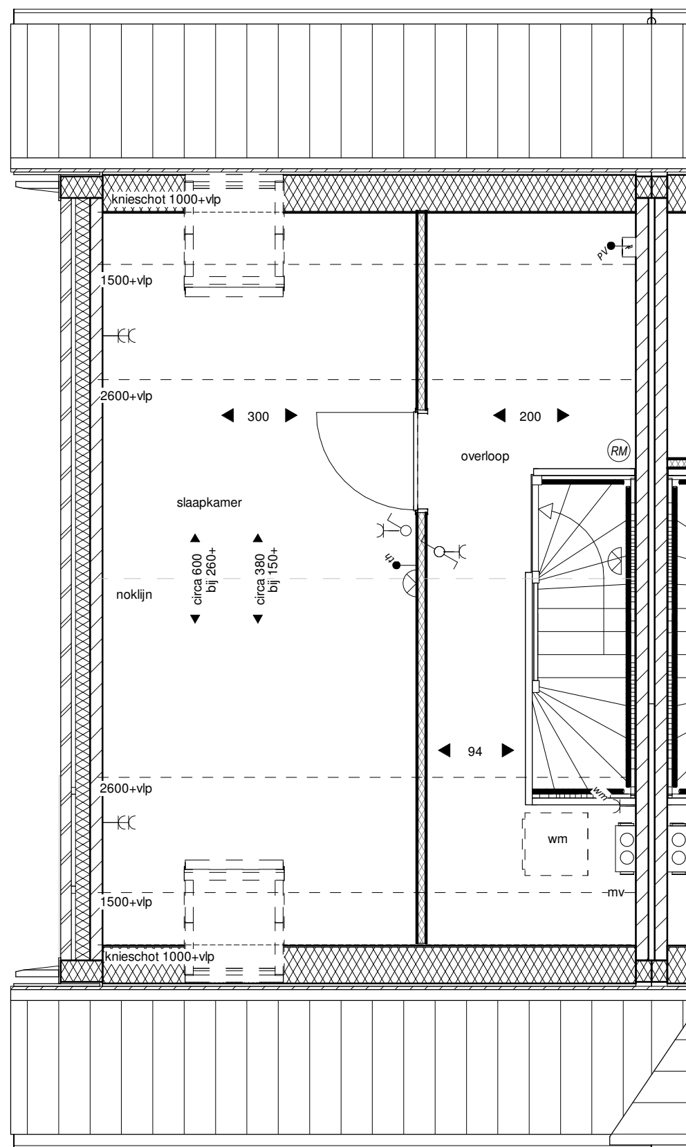
Tweede verdieping
