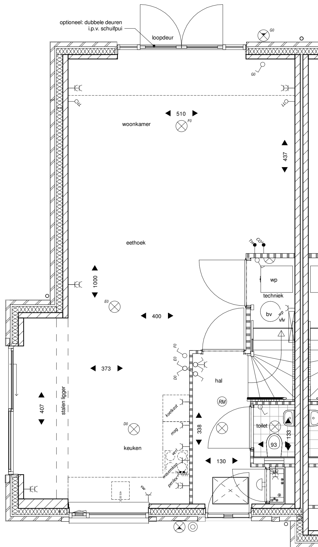
Begane grond
