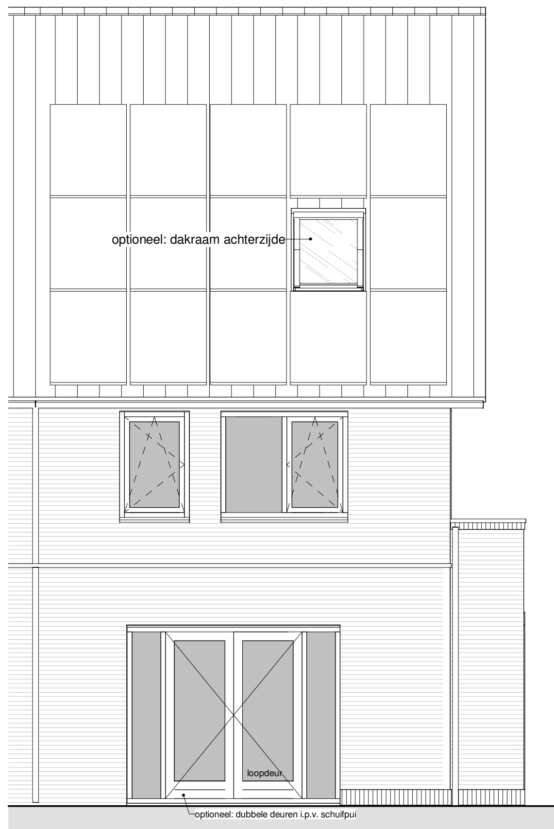
Achtergevel
