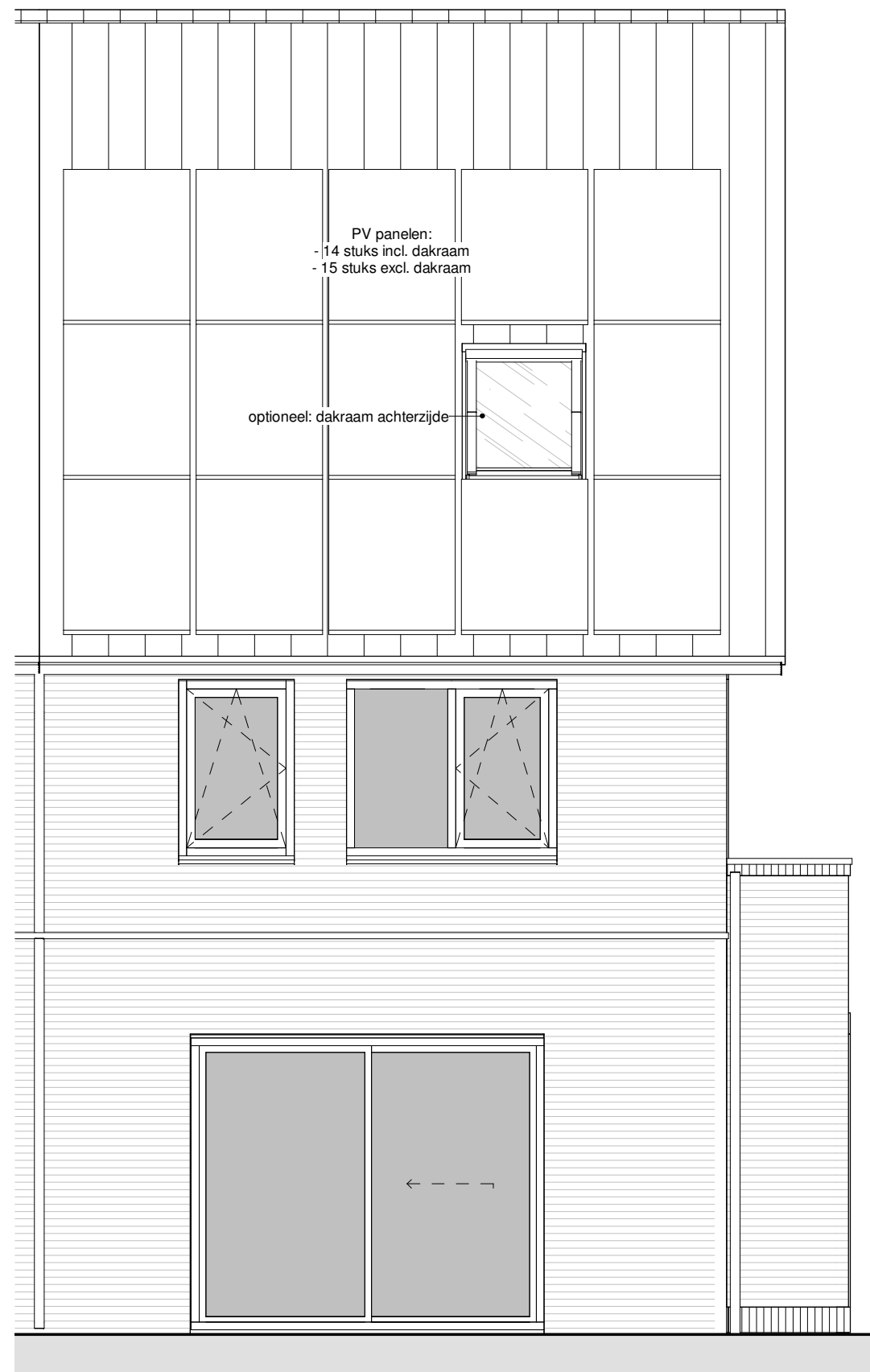
Achtergevel
