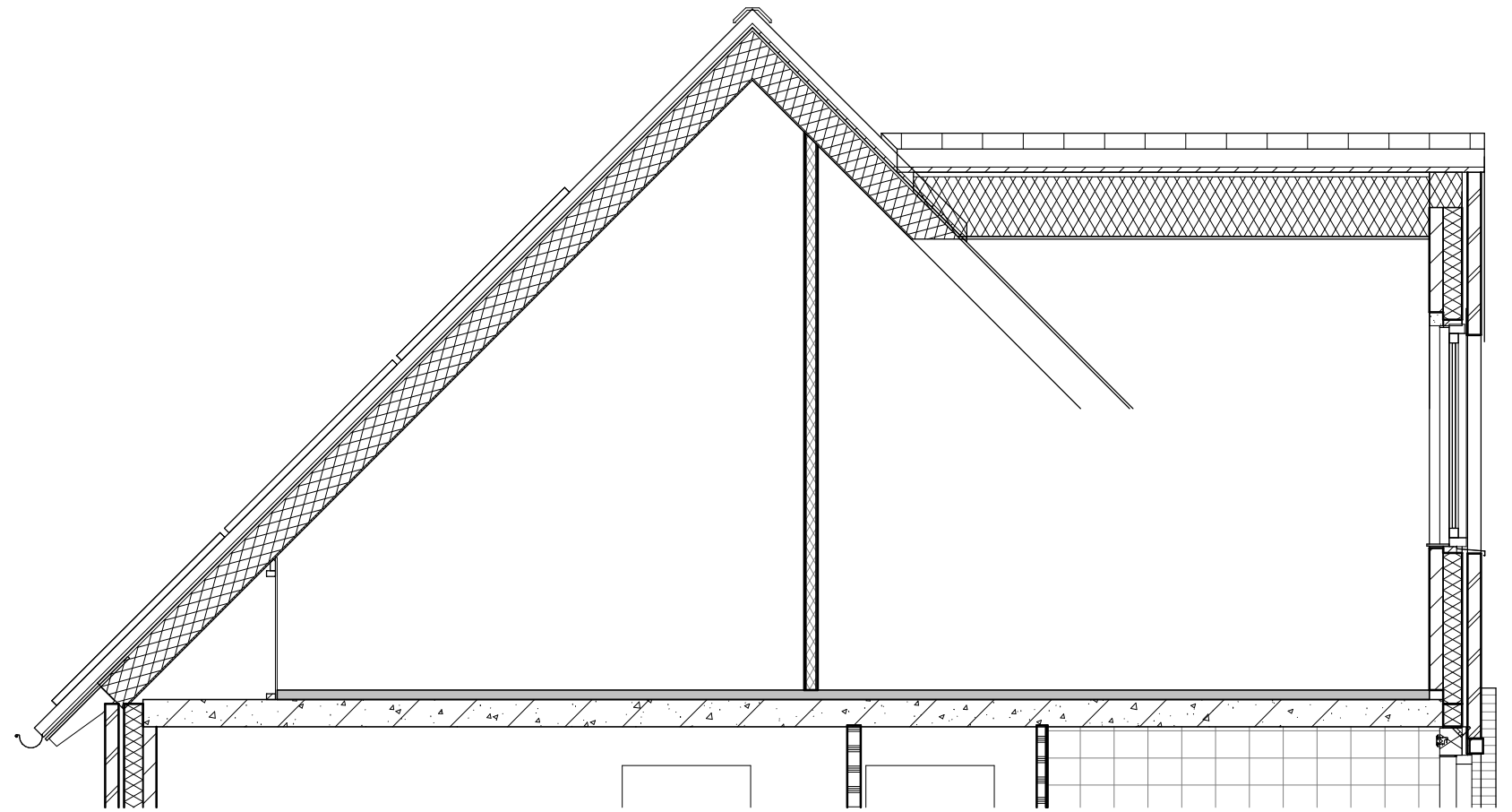
Doorsnede
