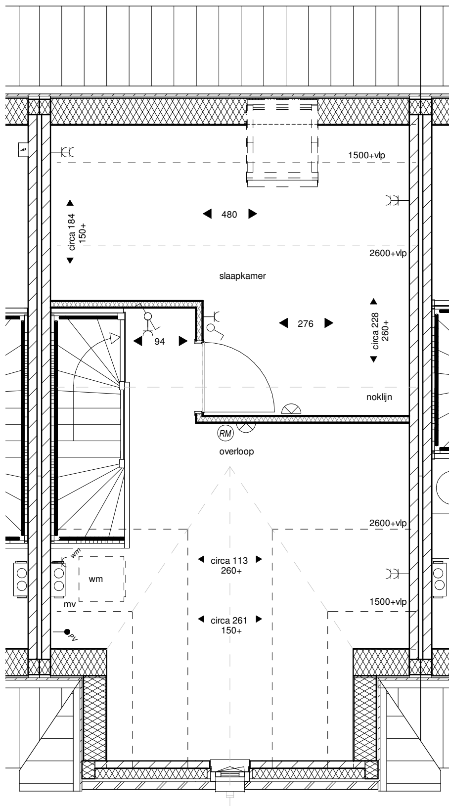
Tweede verdieping
