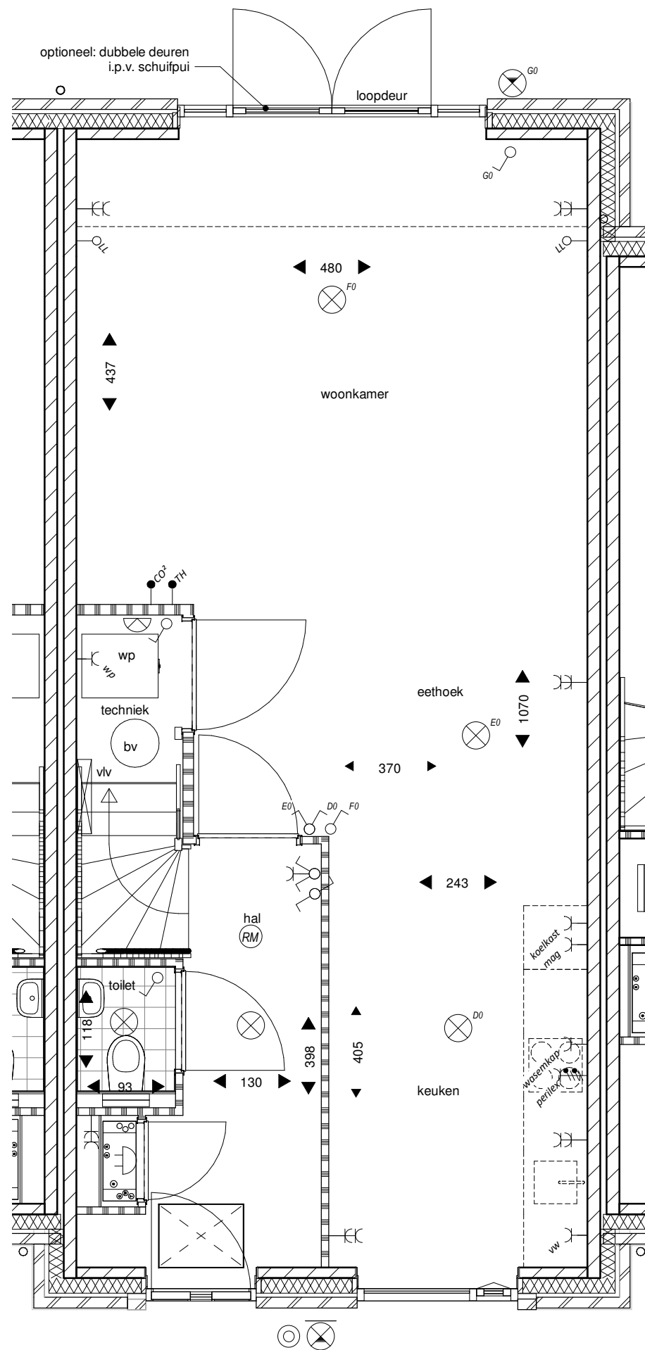
Begane grond
