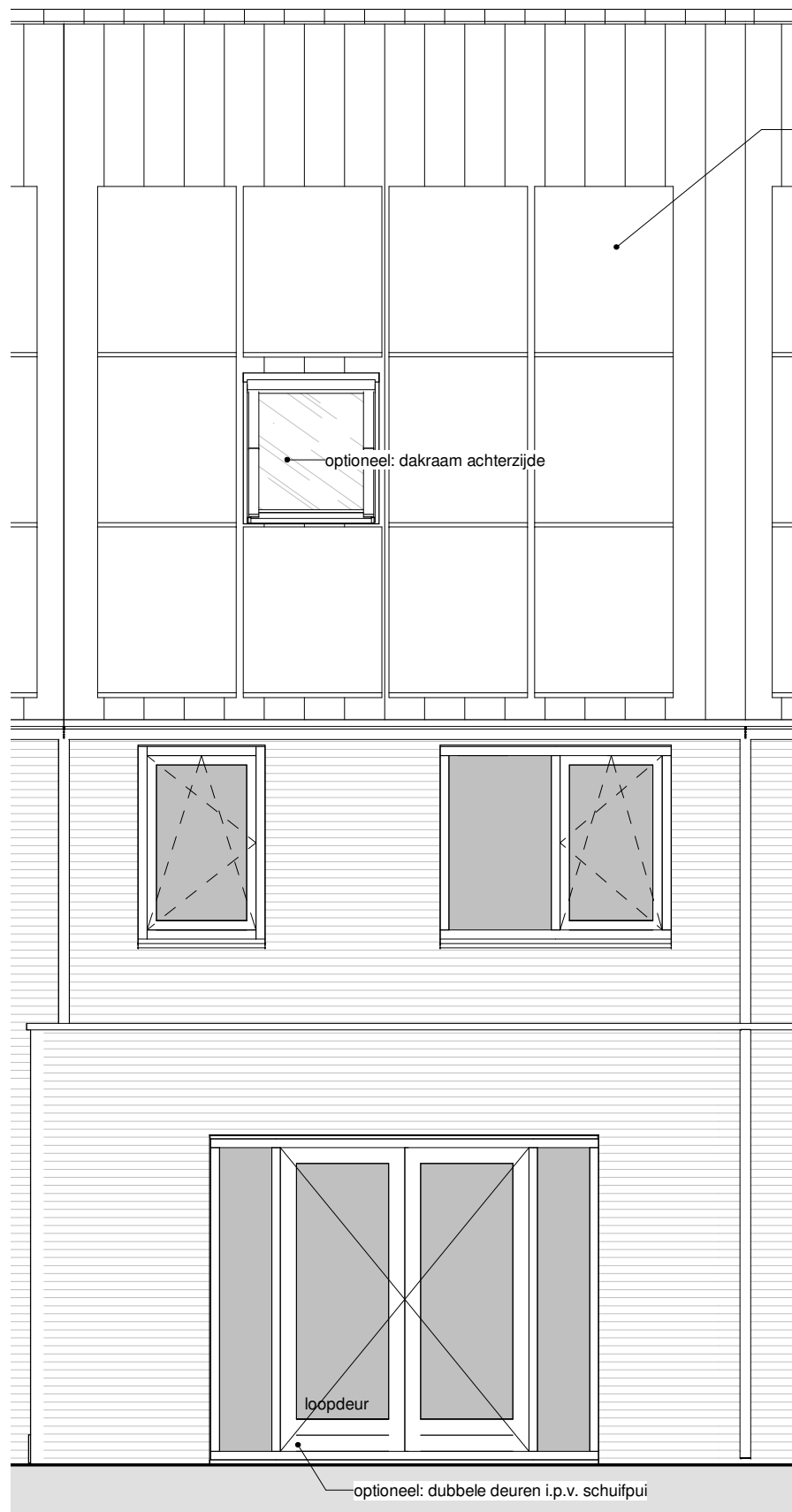
Achtergevel
