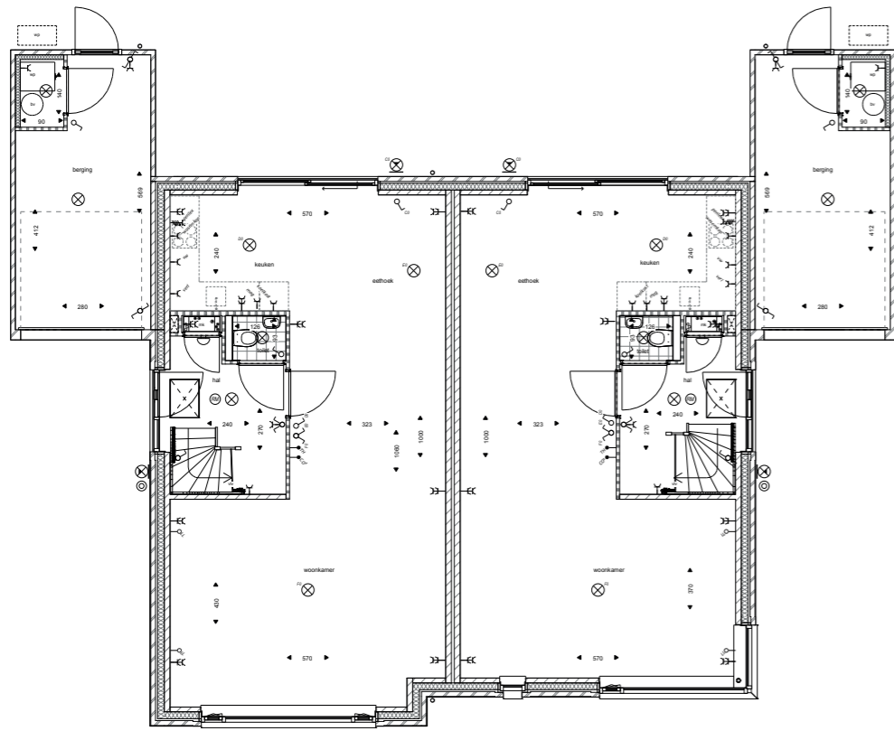
Begane grond
