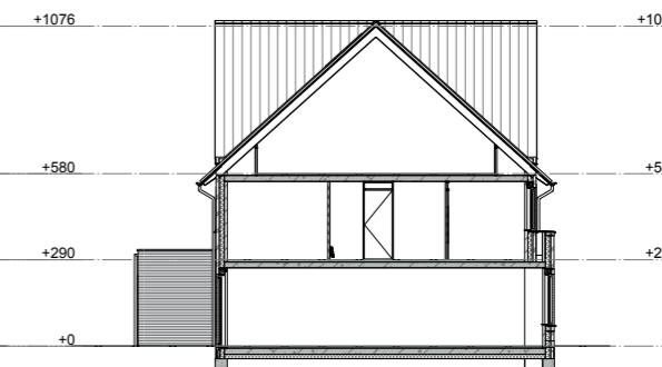
Doorsnede B
