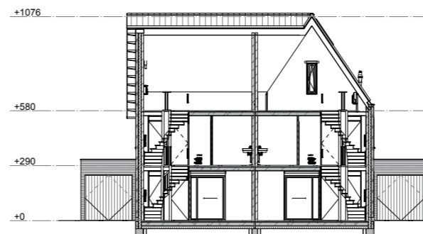
Doorsnede A
