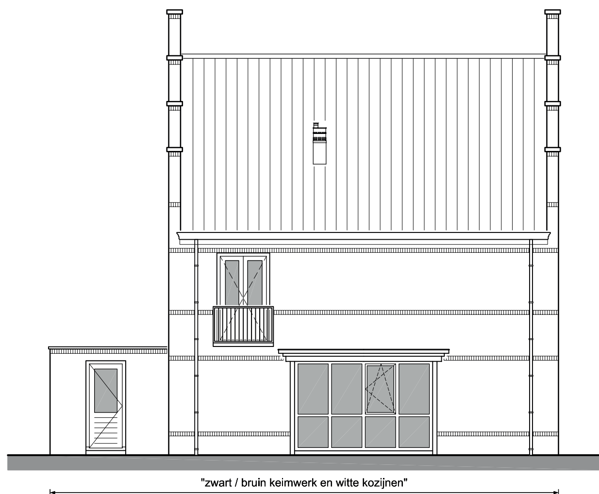
linker zijgevel
