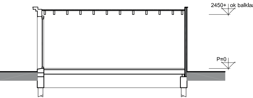
doorsnede bergingen plat dak
