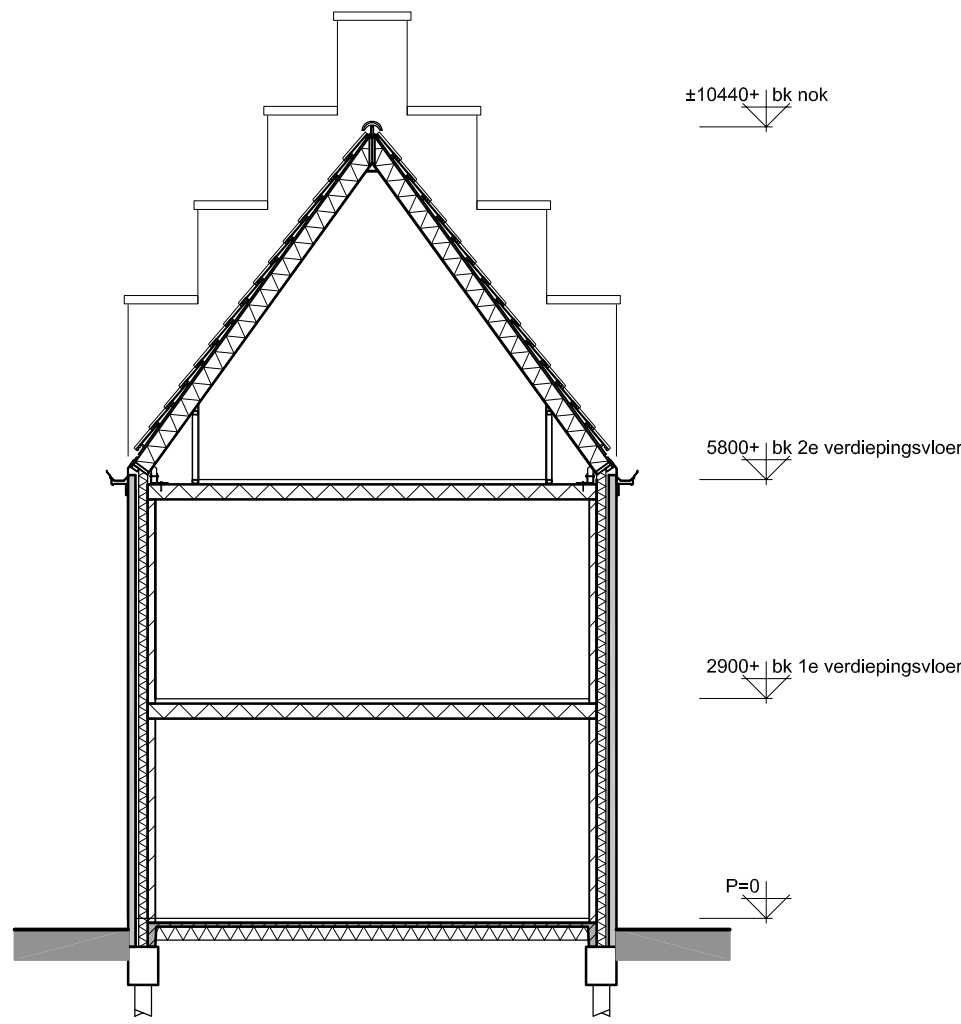
doorsnede bnr. 4 en 5
