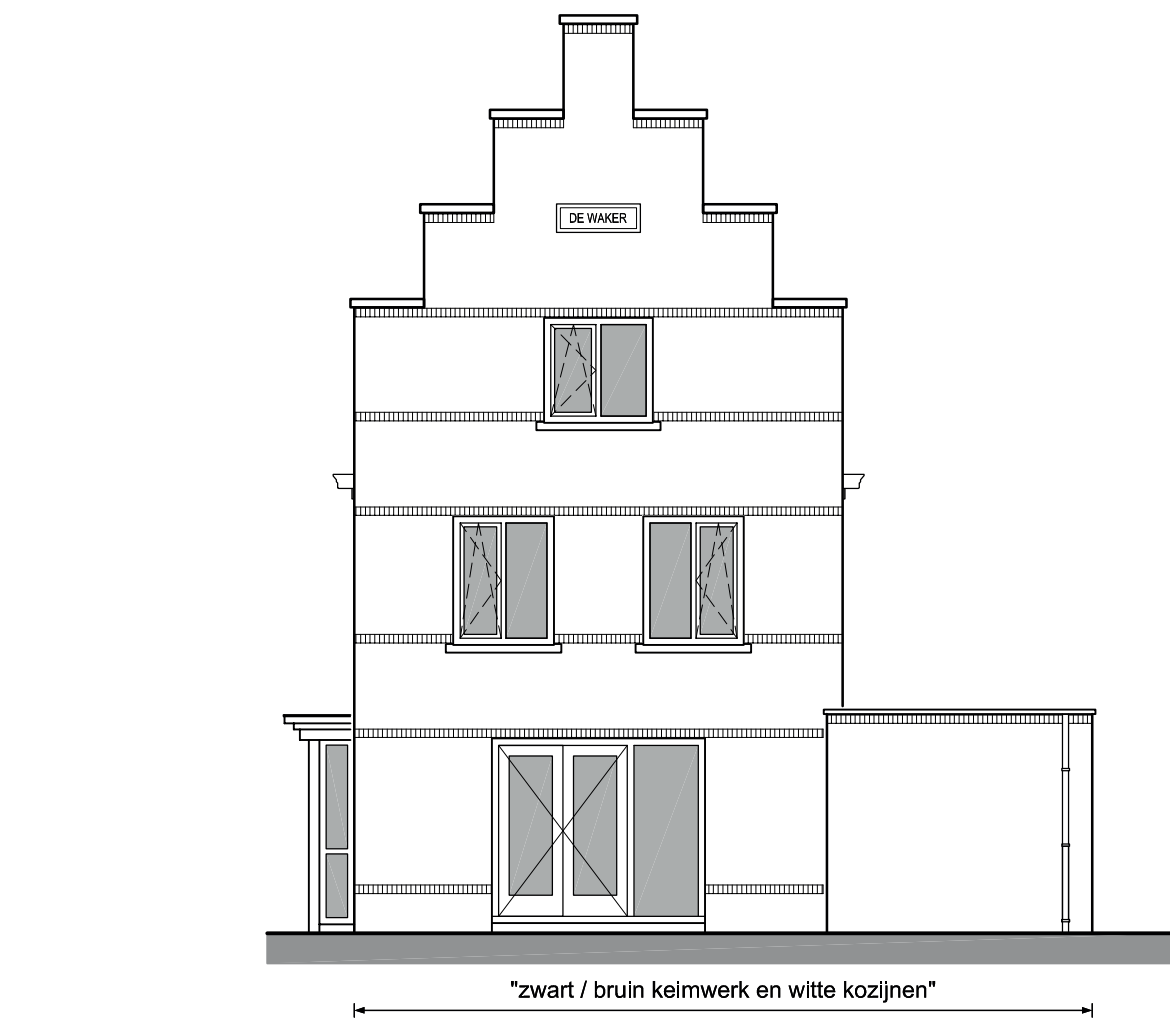
achtergevel
