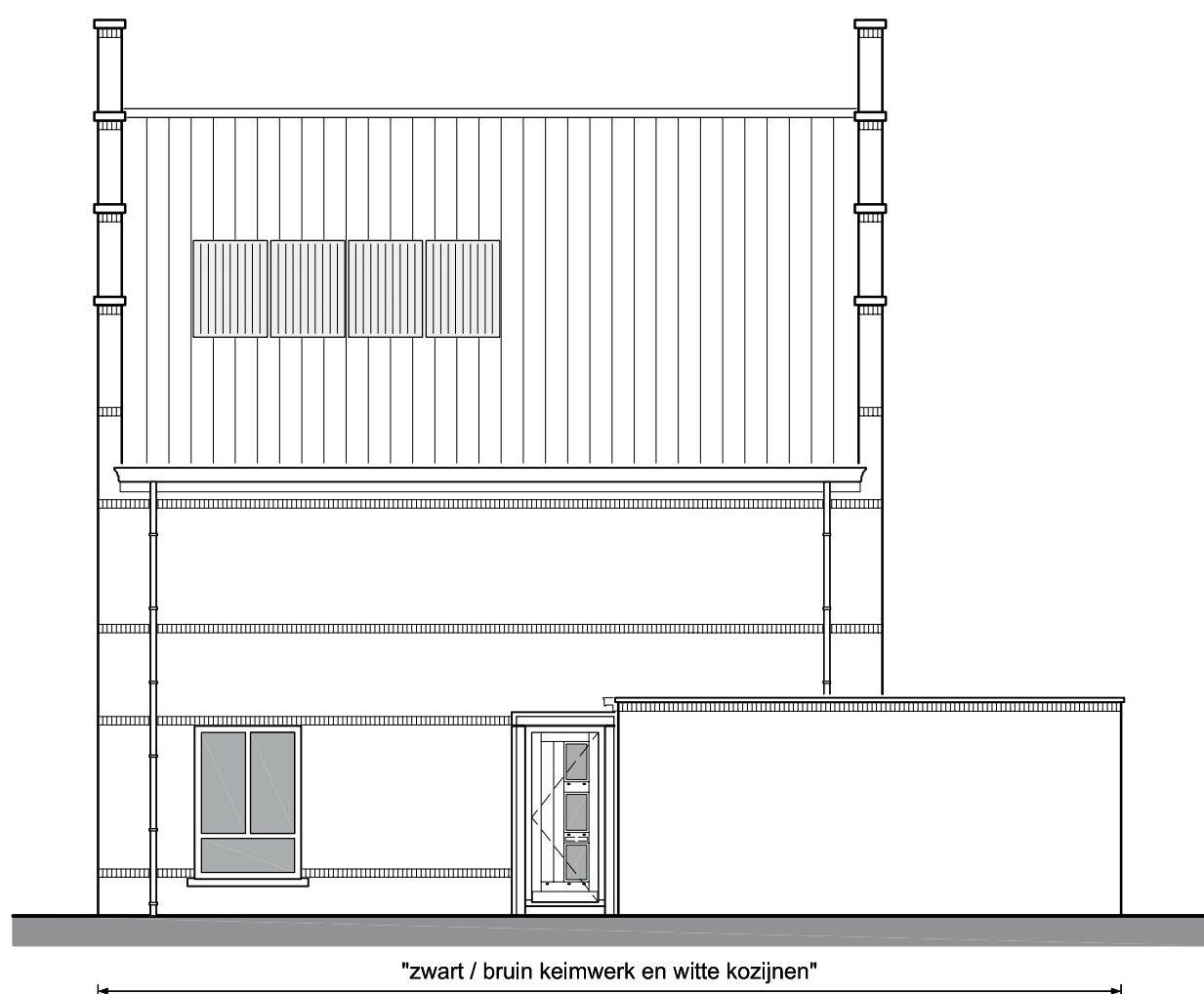
rechter zijgevel
