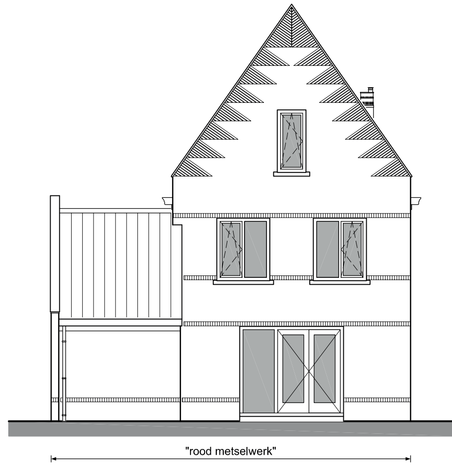
achtergevel
