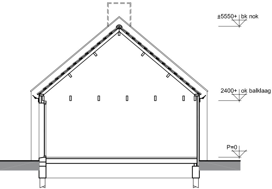
doorsnede bergingen
