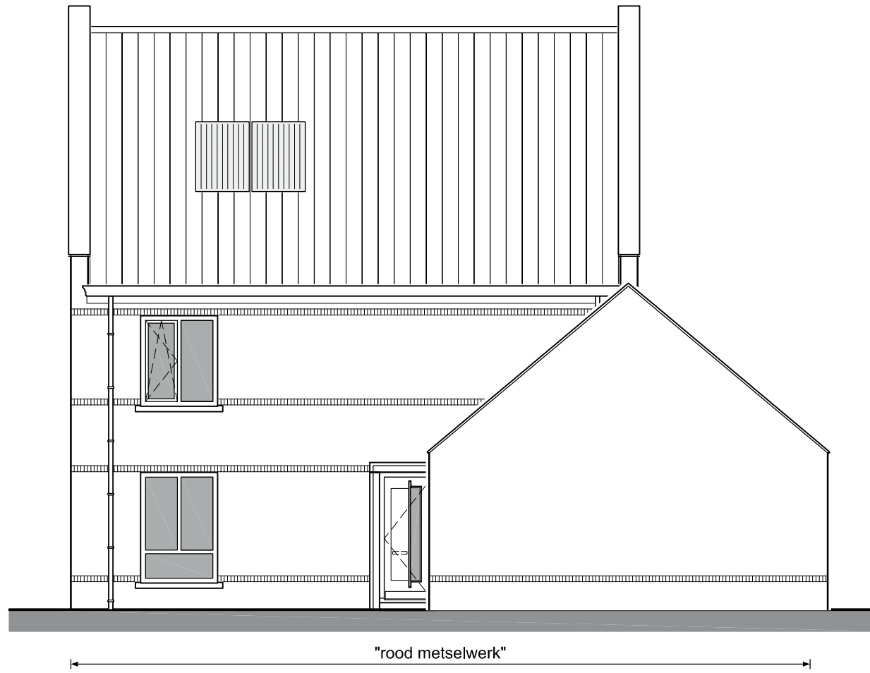
rechter zijgevel
