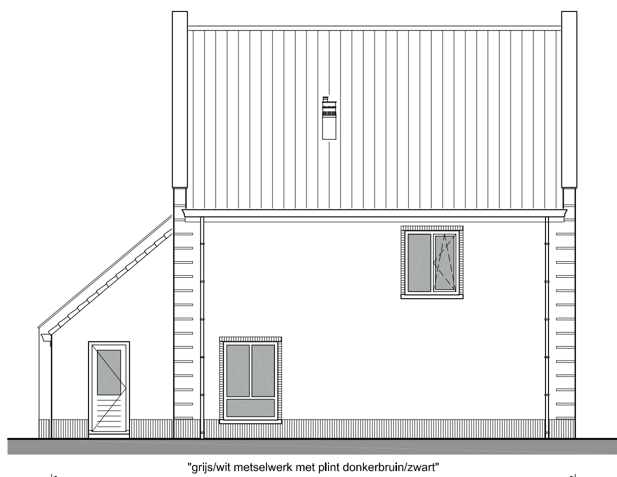
linker zijgevel
