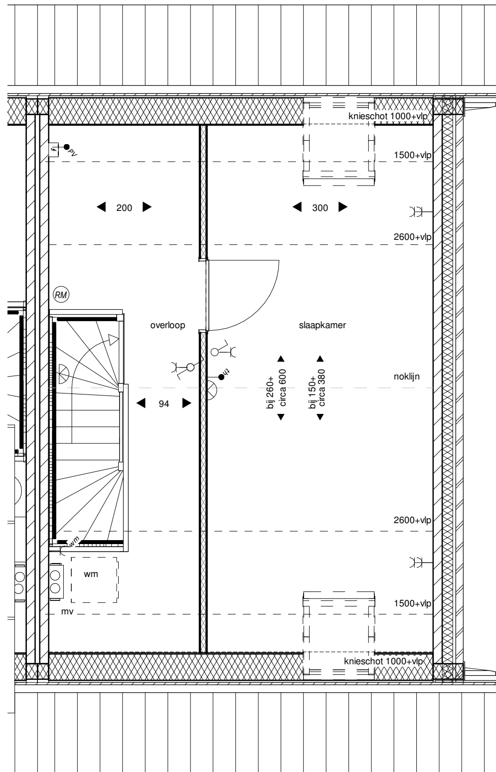
Tweede verdieping
