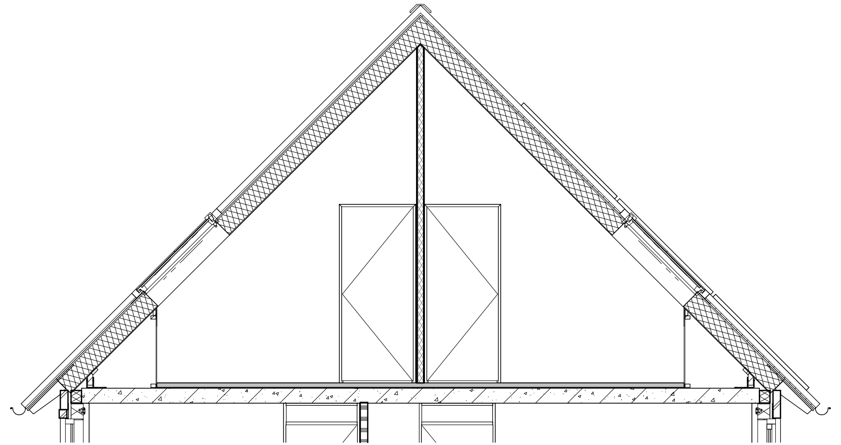
Doorsnede
