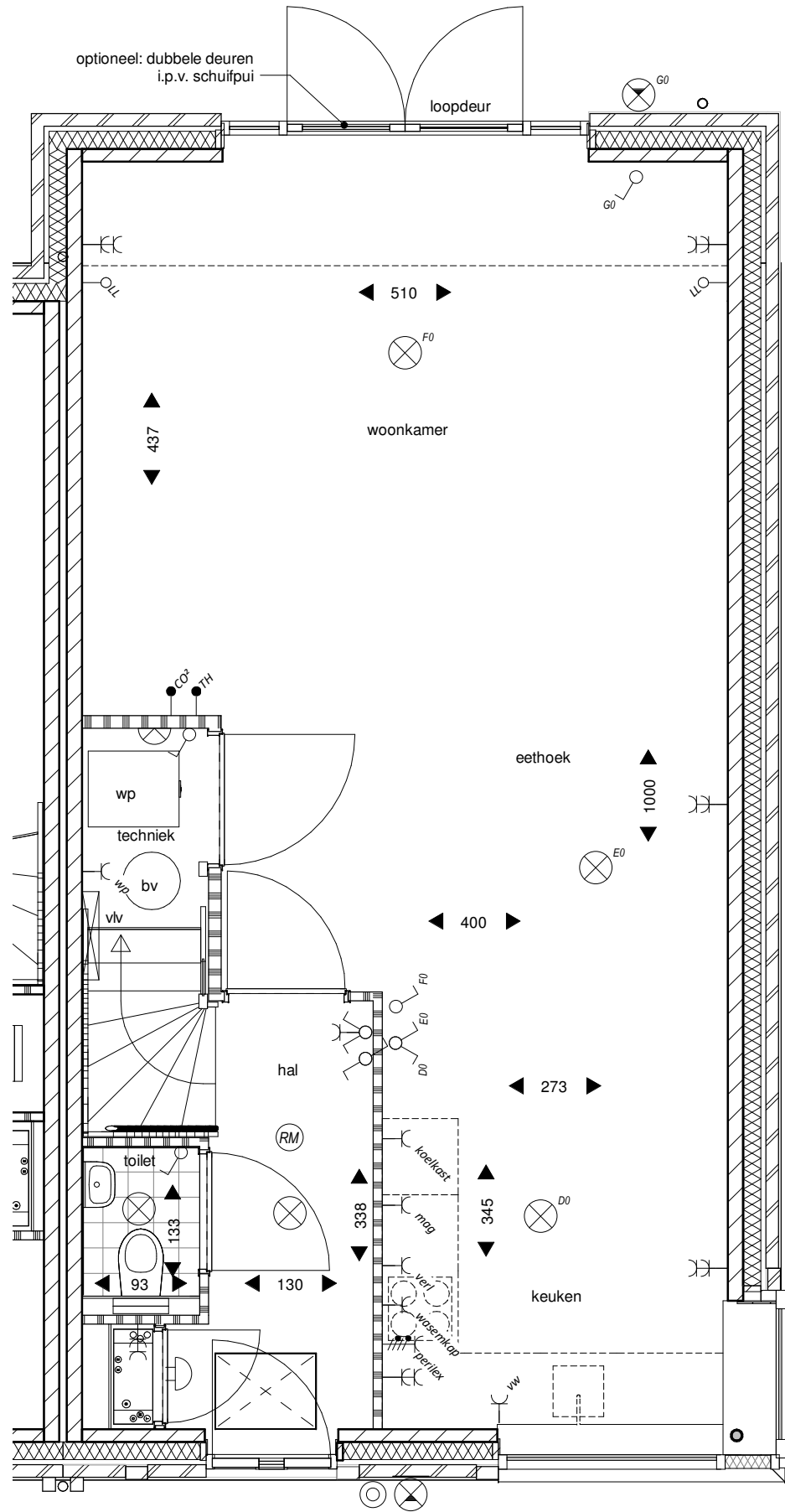
Begane grond
