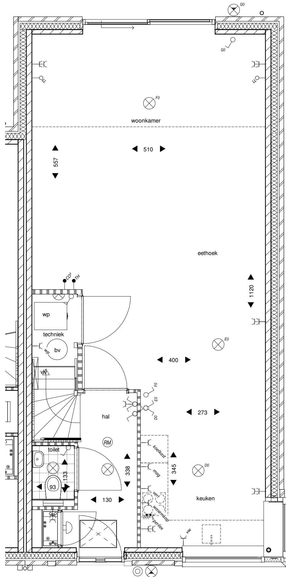
Begane grond
