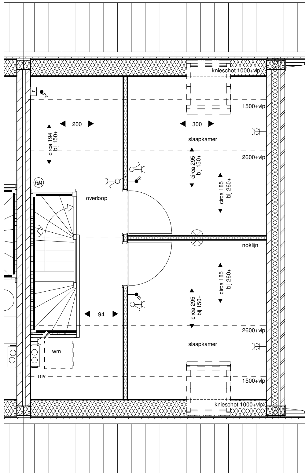
Tweede verdieping
