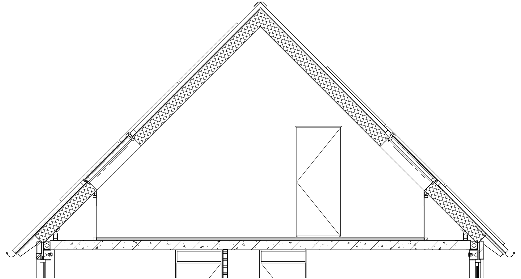
Doorsnede
