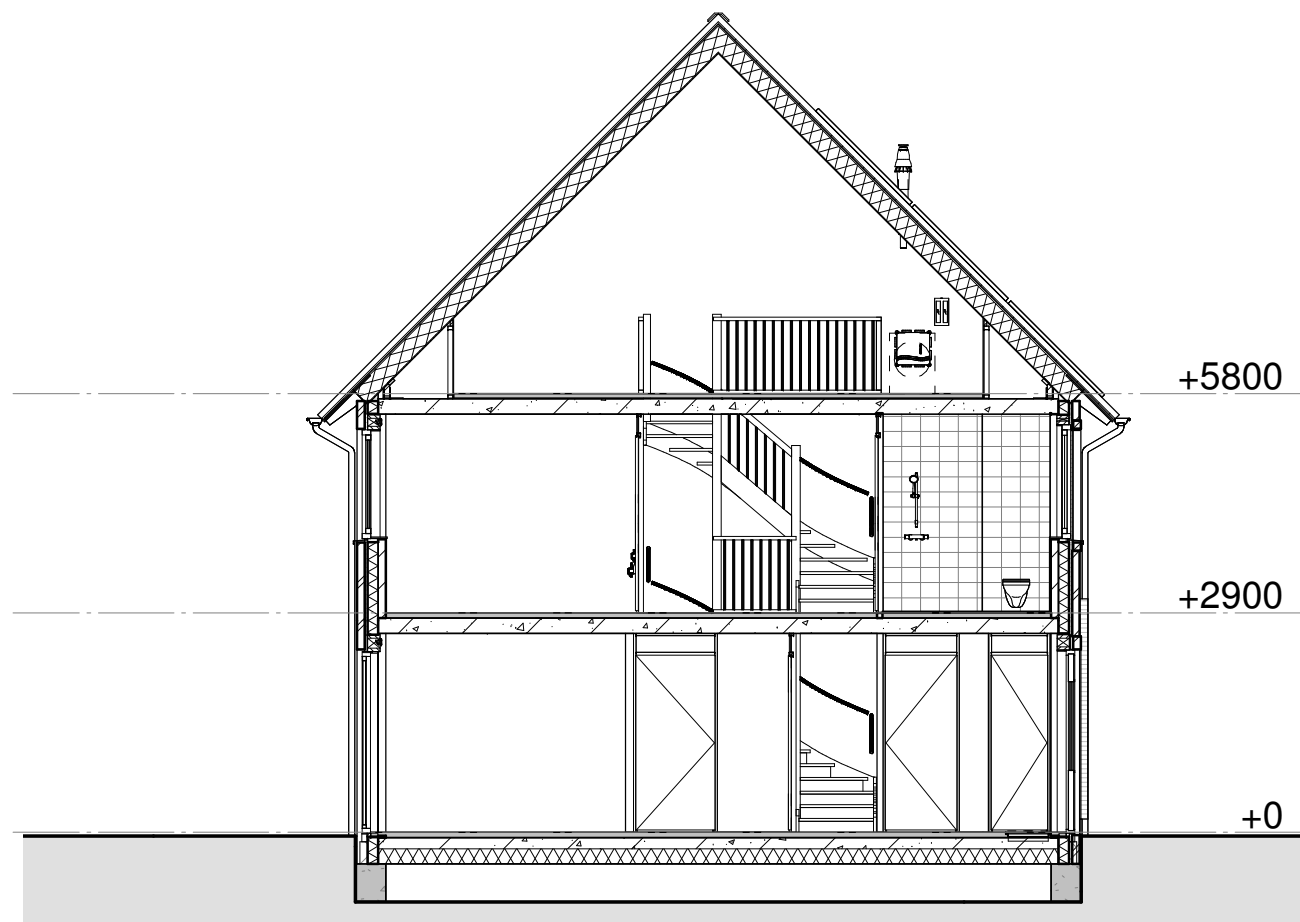
Doorsnede 17-A
