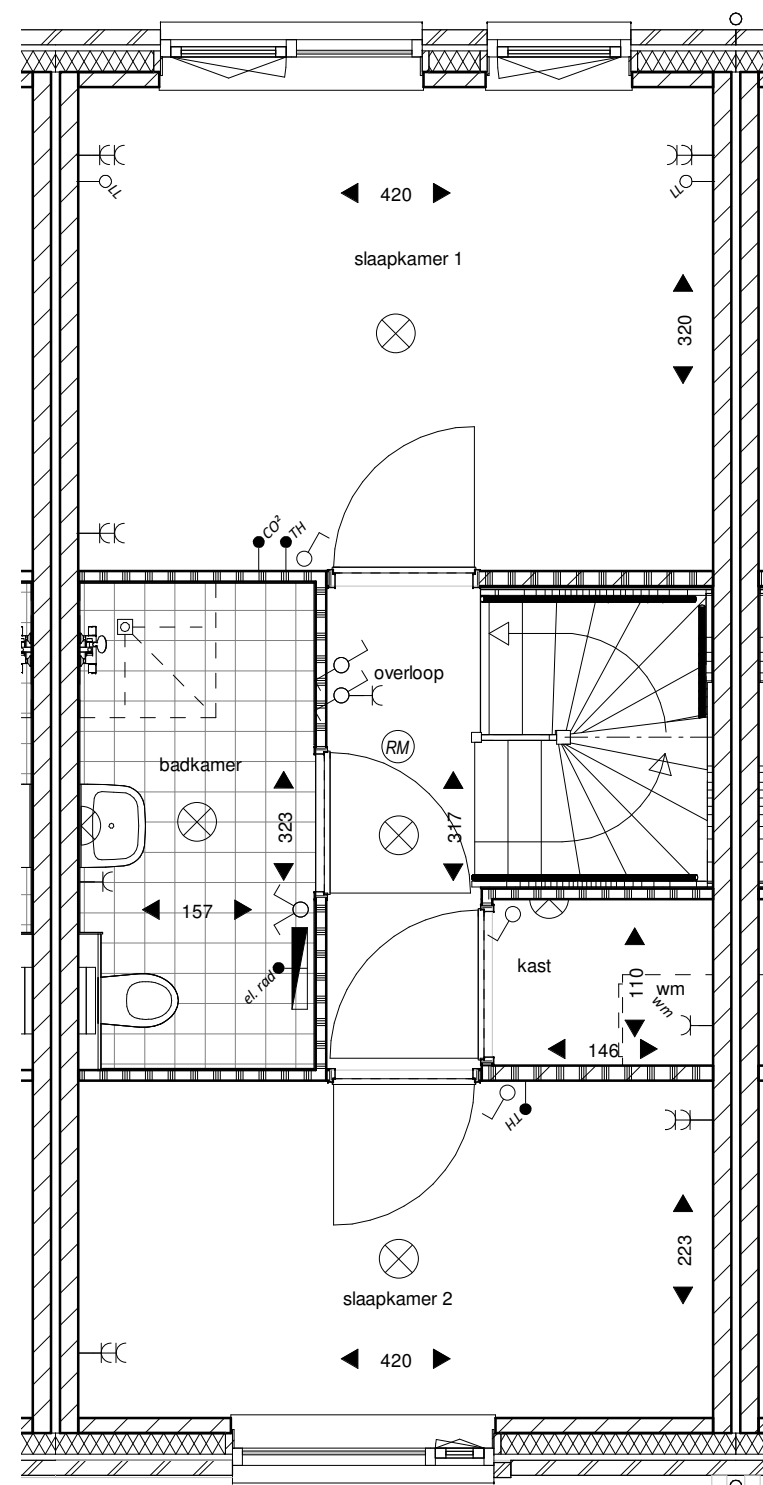
eerste verdieping
