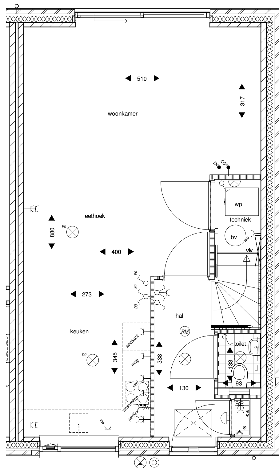
begane grond
