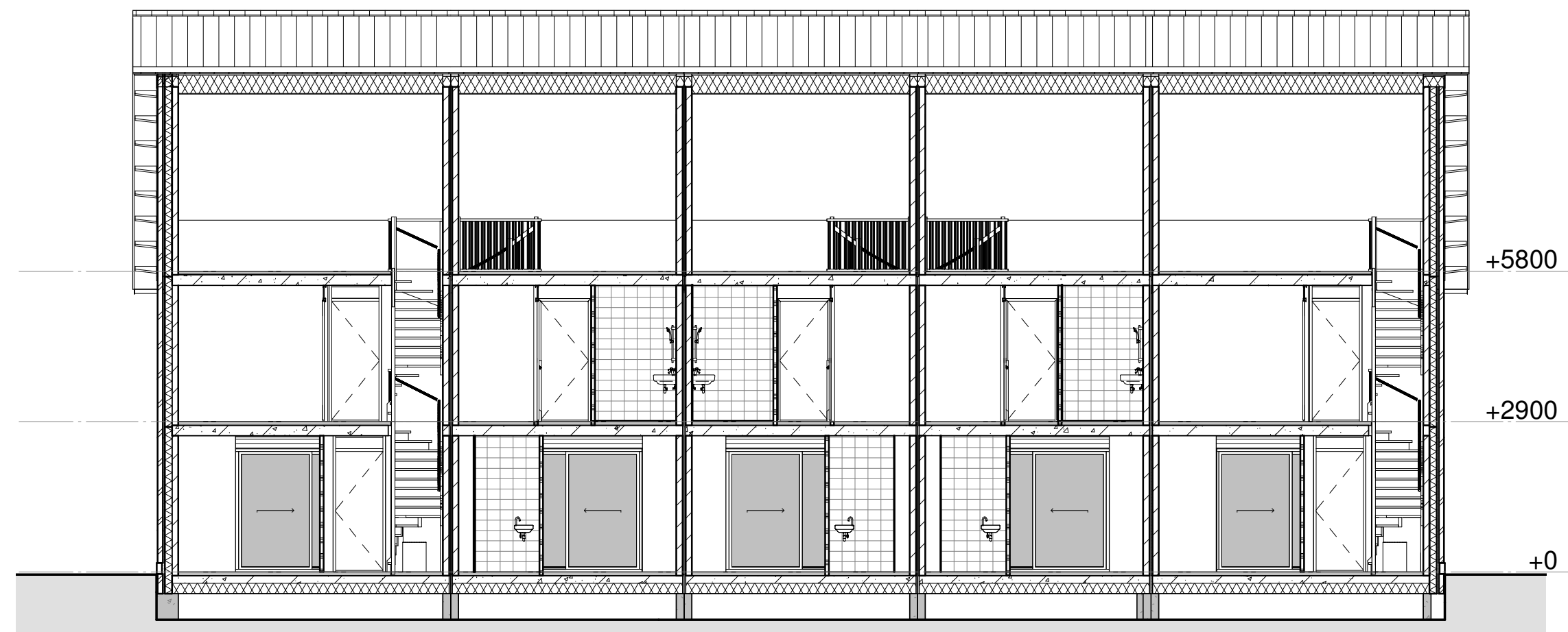
Doorsnede 17-B
