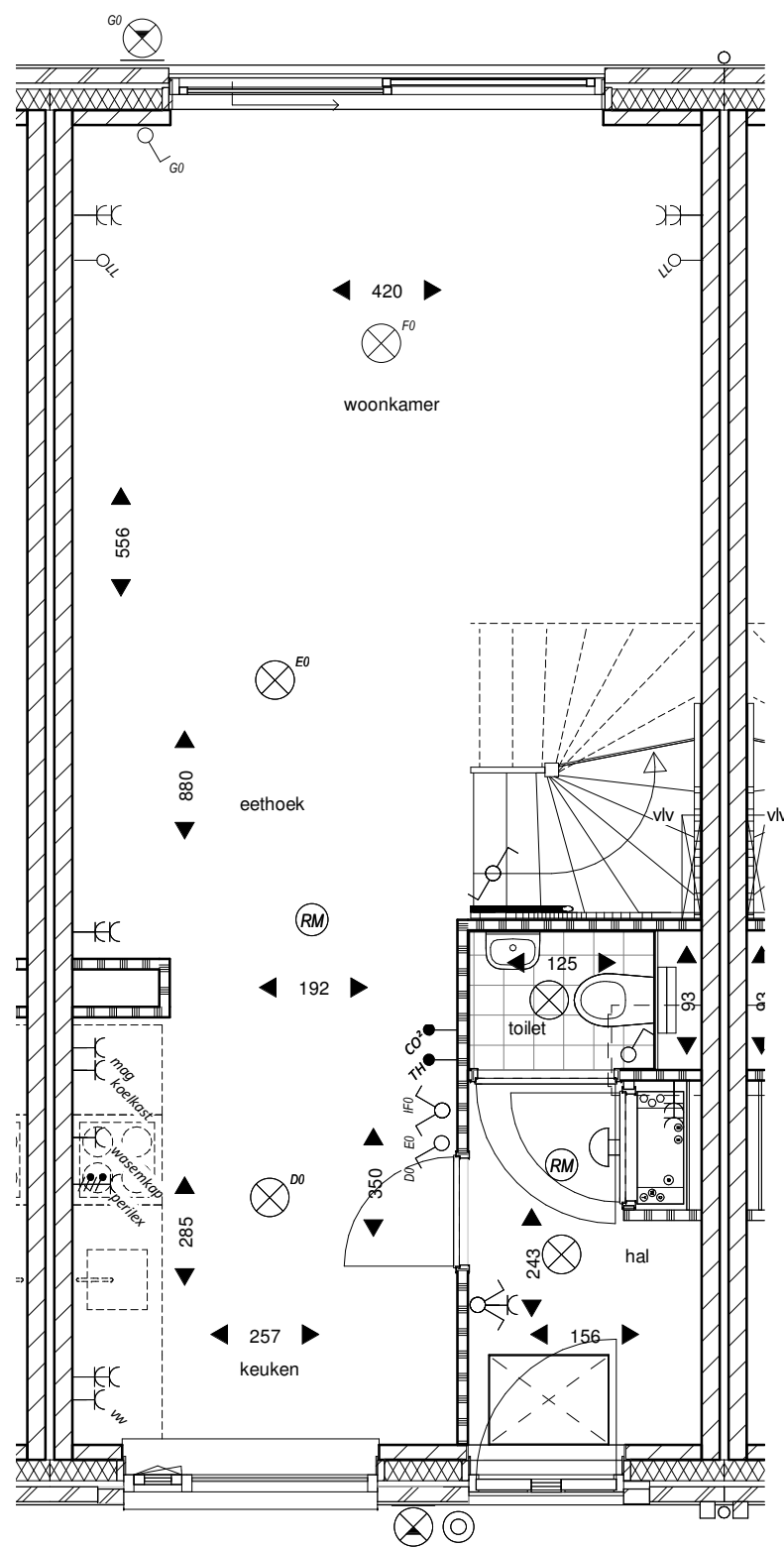
begane grond
