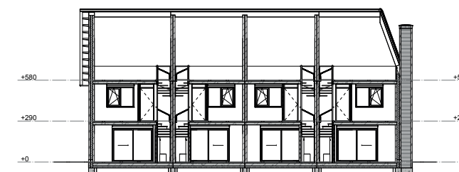
Doorsnede B
