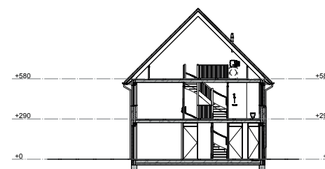
Doorsnede A
