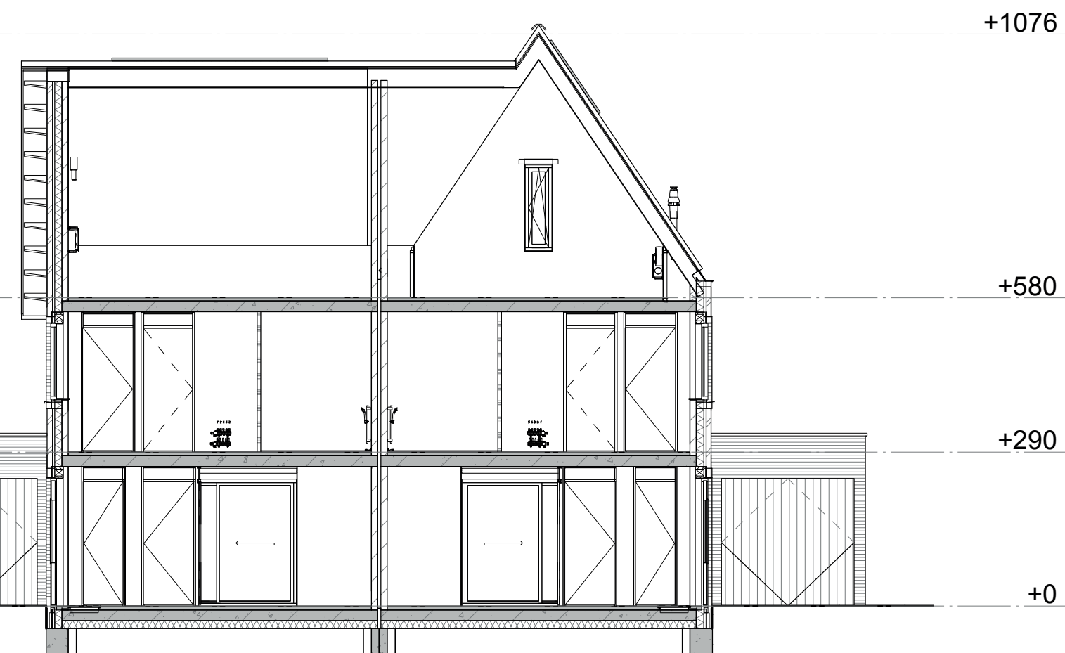
Doorsnede B
