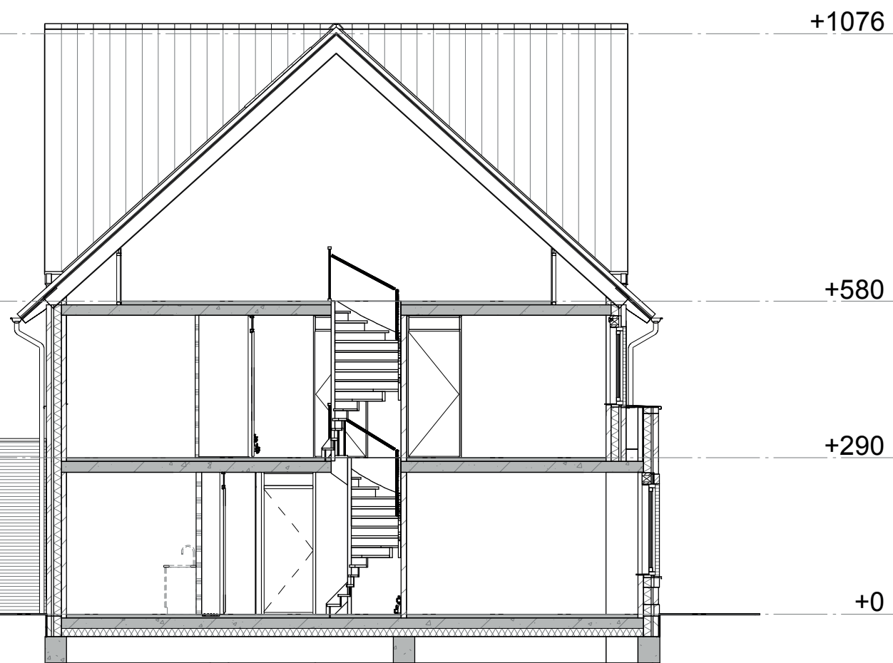
Doorsnede A
