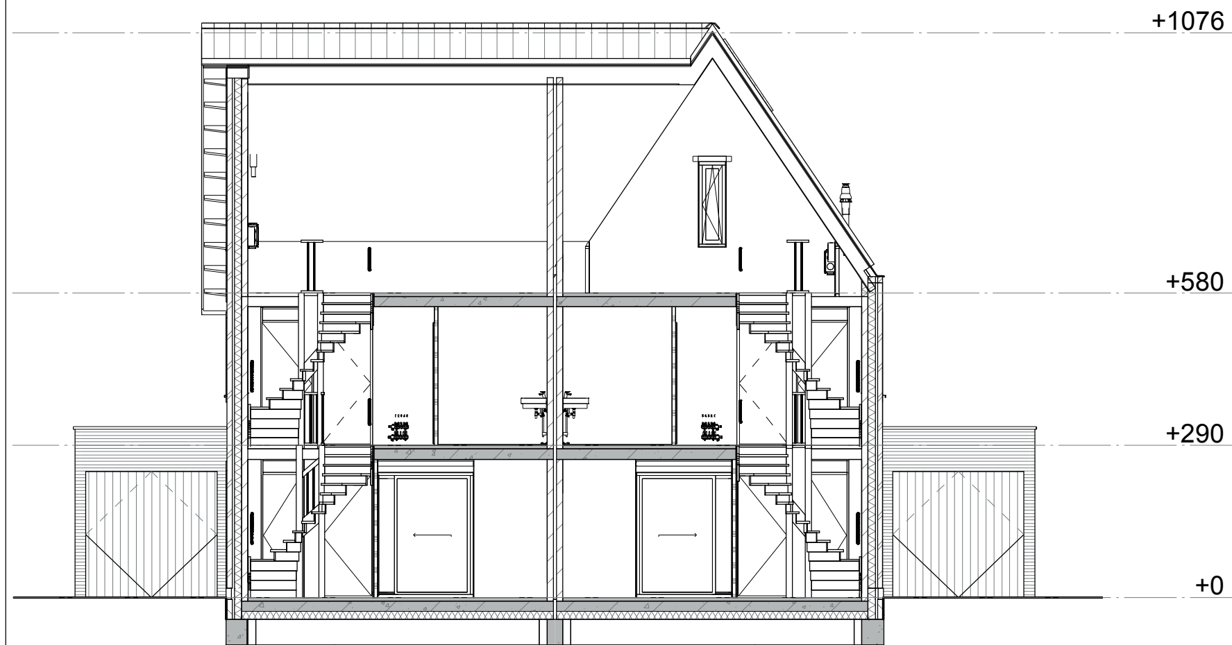
Doorsnede A
