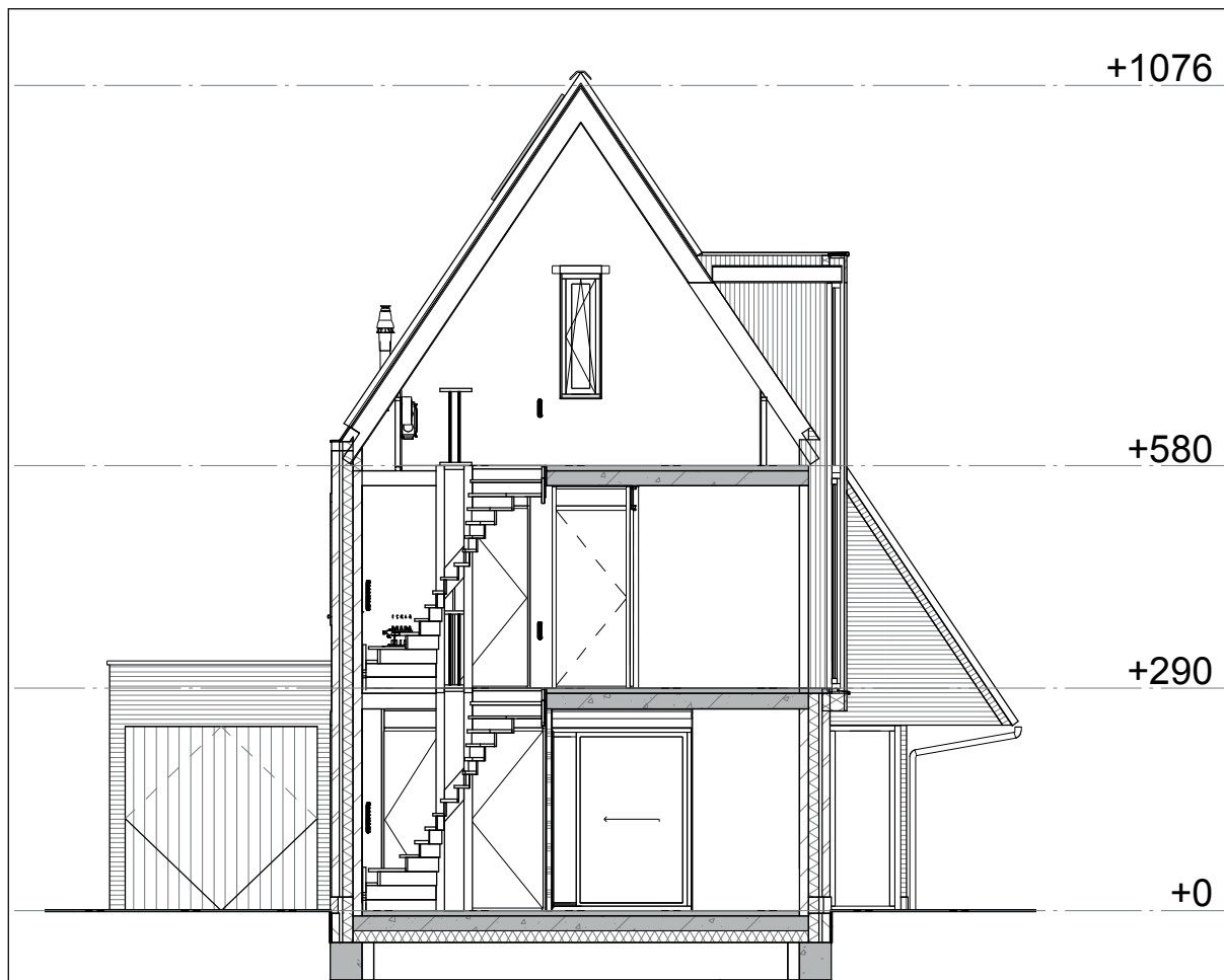
Doorsnede A
