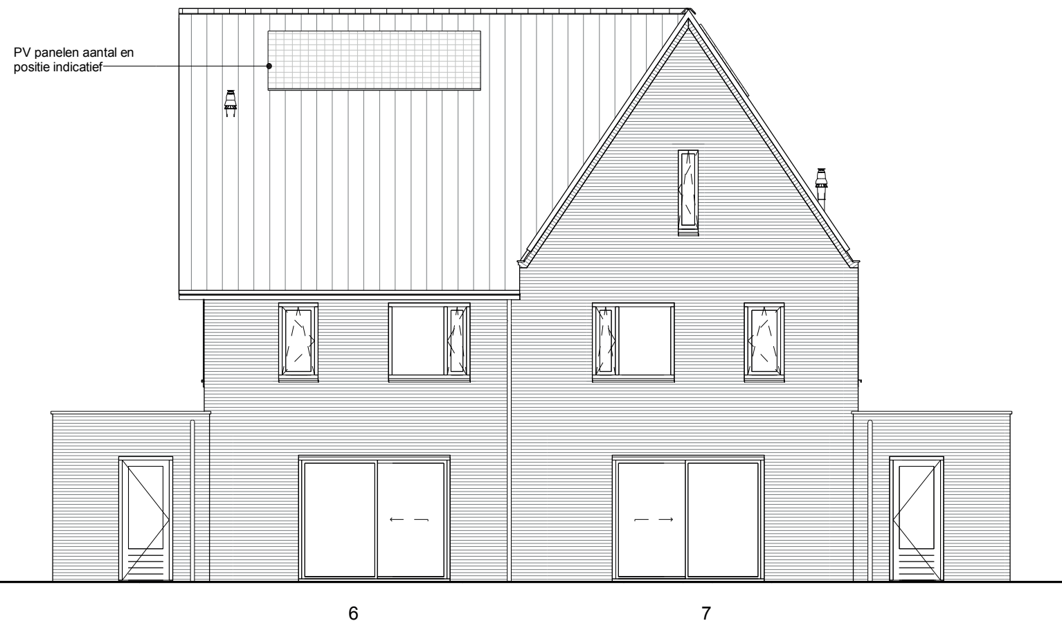
Achtergevel
