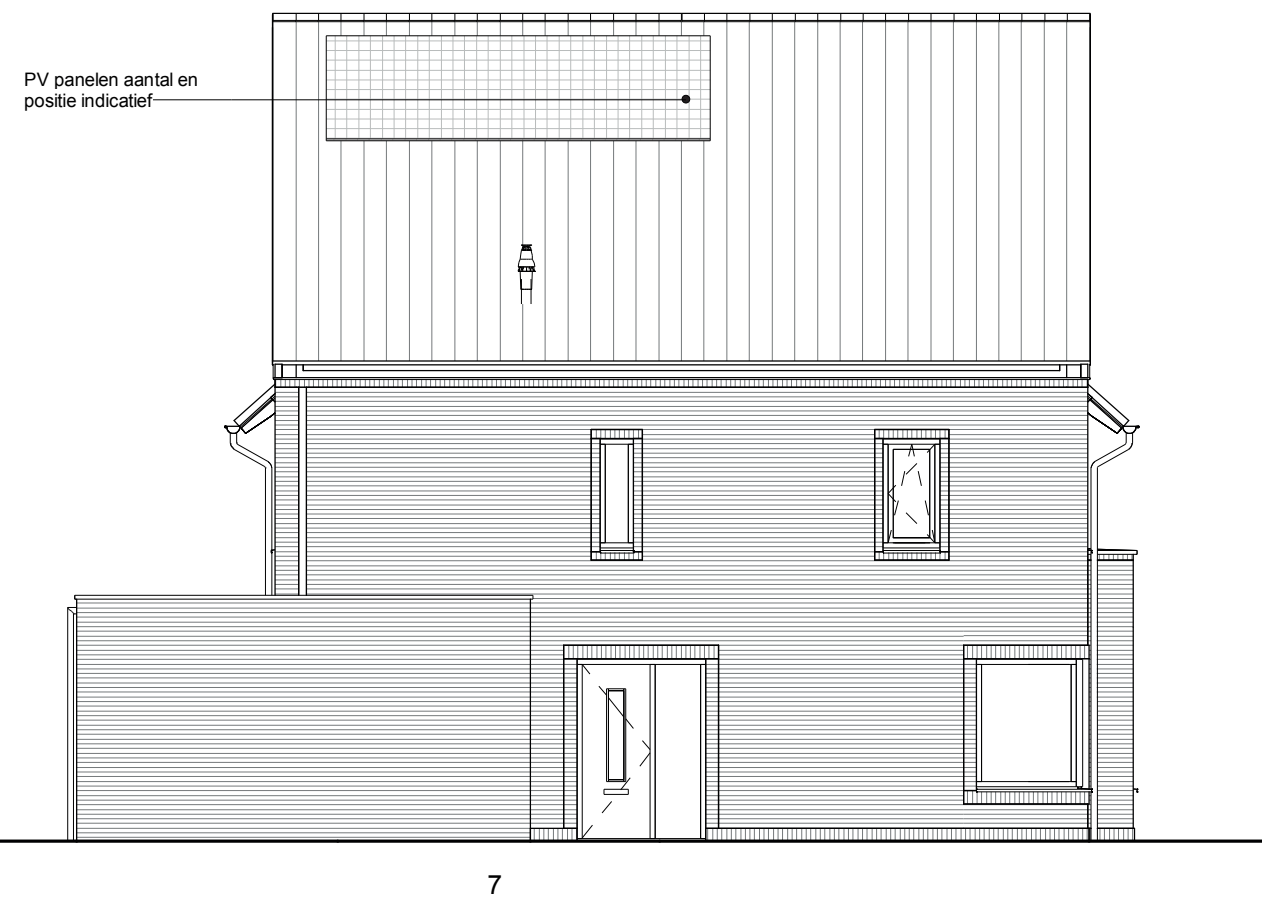
Linkergevel
