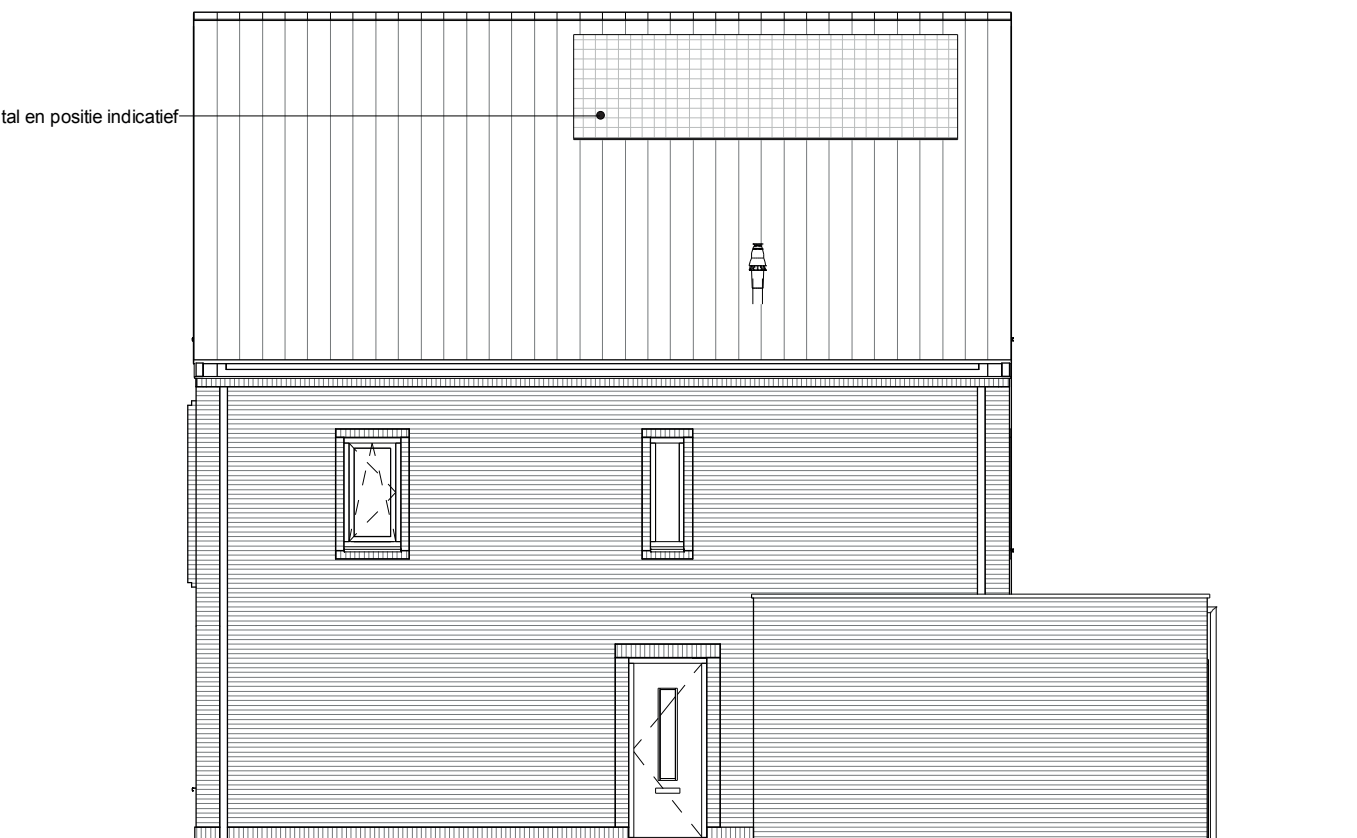
Rechtergevel
