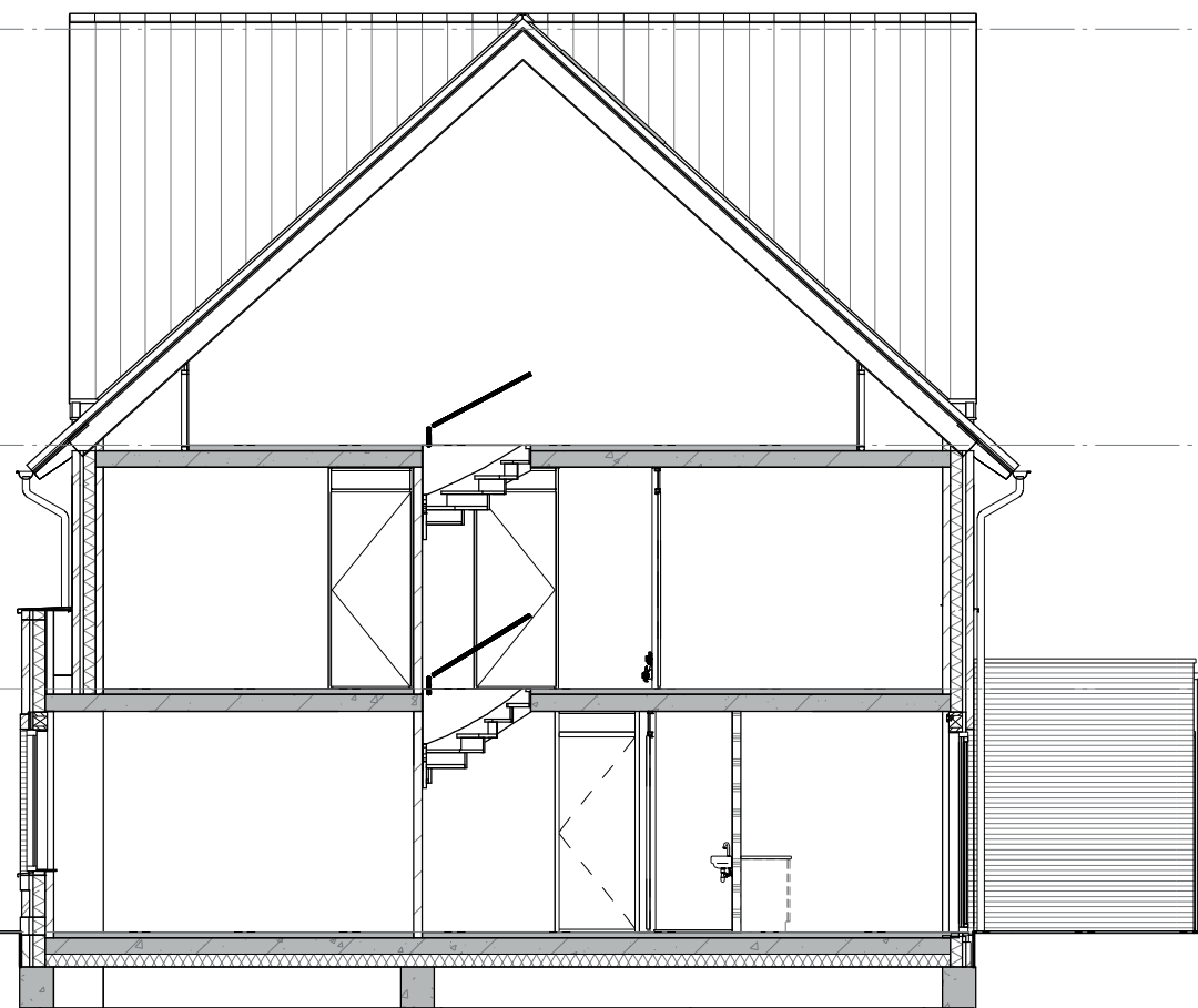
Doorsnede A
