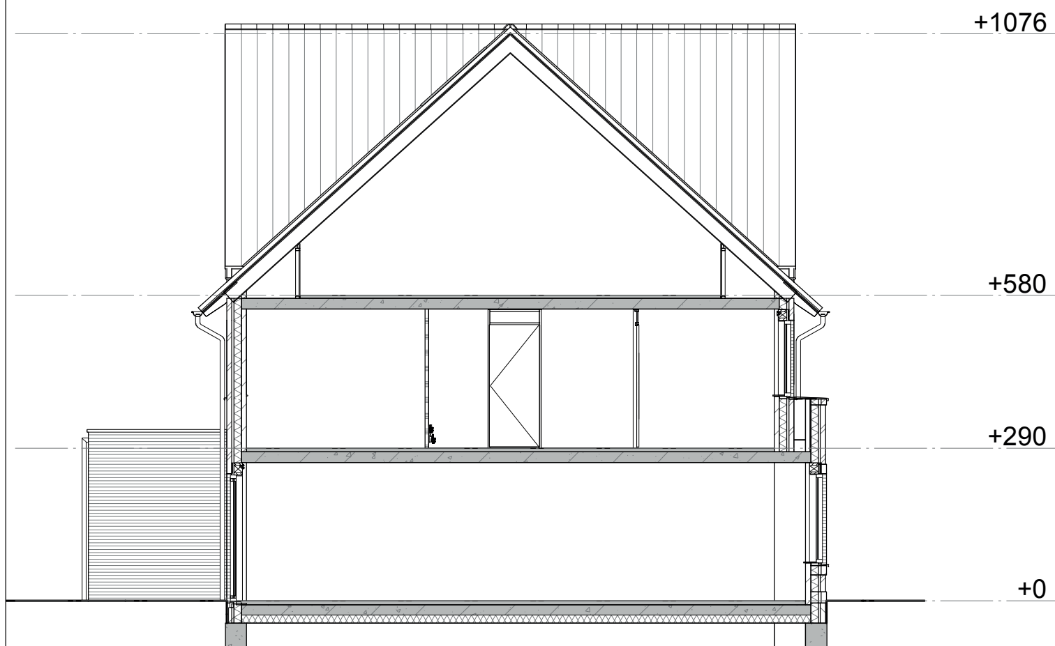
Doorsnede B
