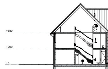
Doorsnede A
