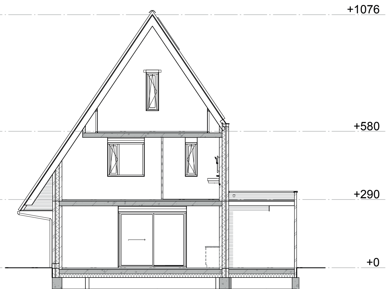
Doorsnede A
