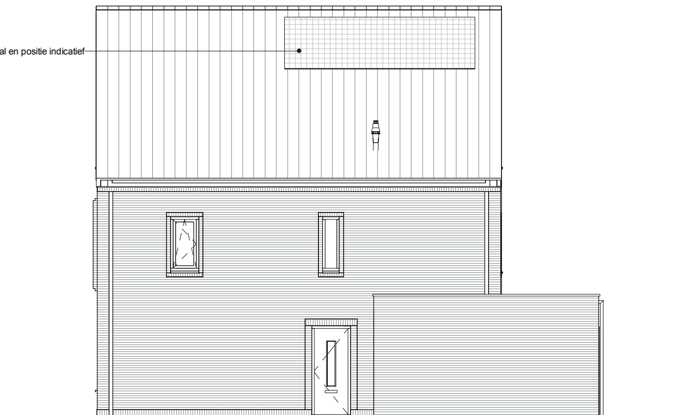
Rechtergevel
