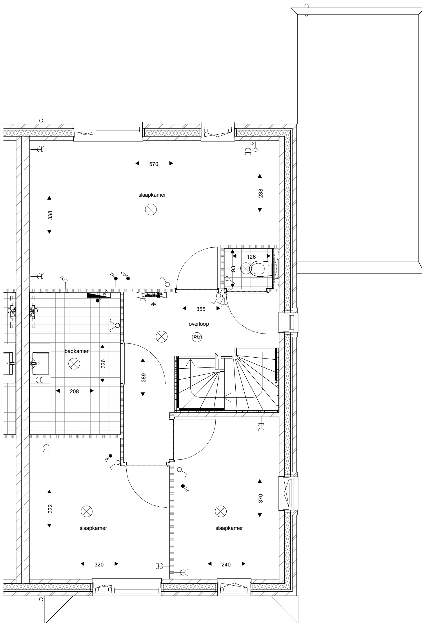
Eerste verdieping bouwnr 38
