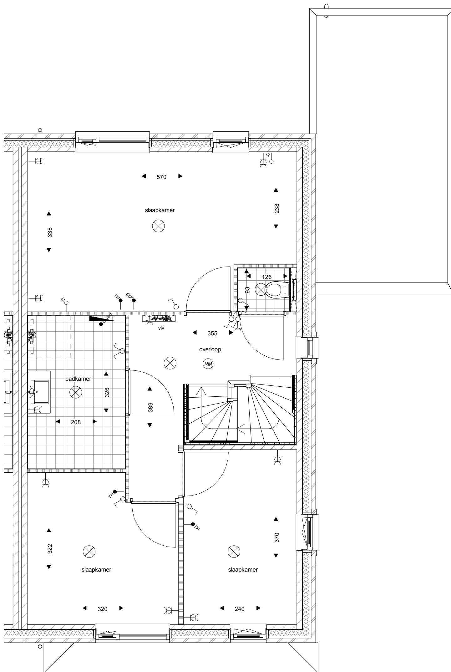
Eerste verdieping bouwnr 42
