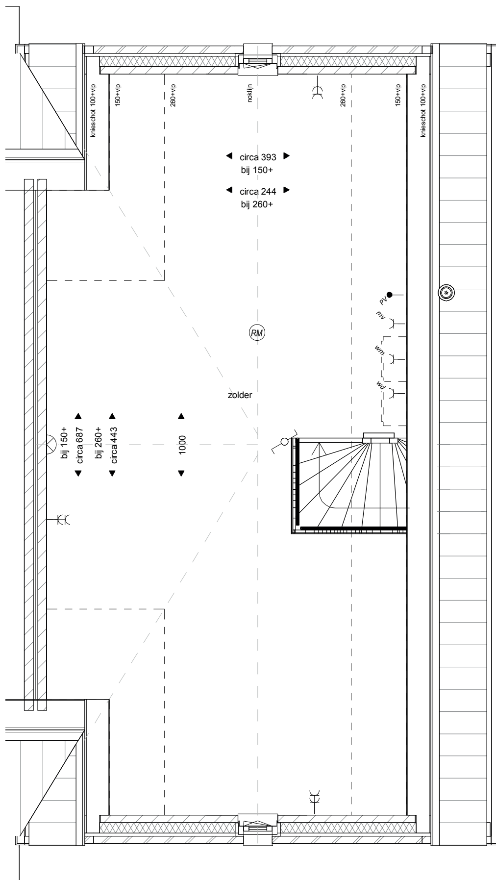
Tweede verdieping bouwnr 40
