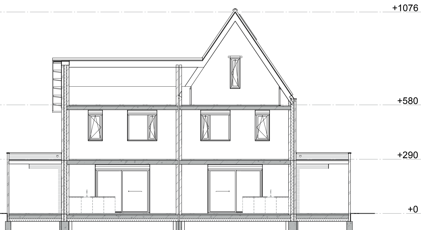
Doorsnede B
