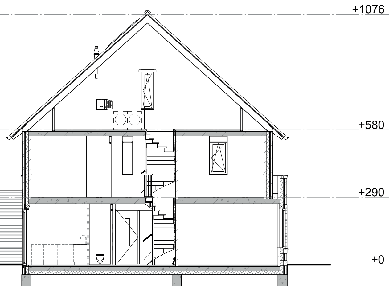
Doorsnede A
