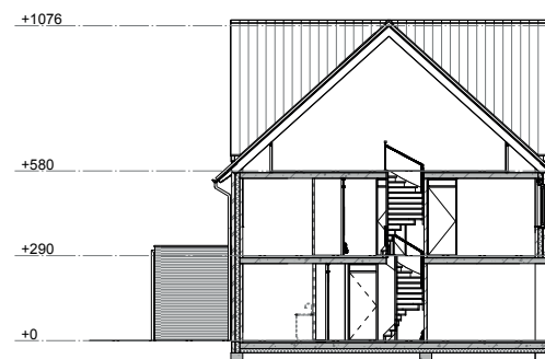
Doorsnede A
