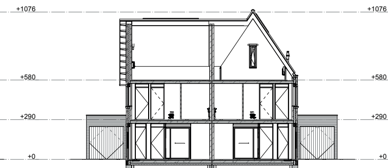
Doorsnede B
