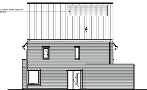
Rechtergevel
