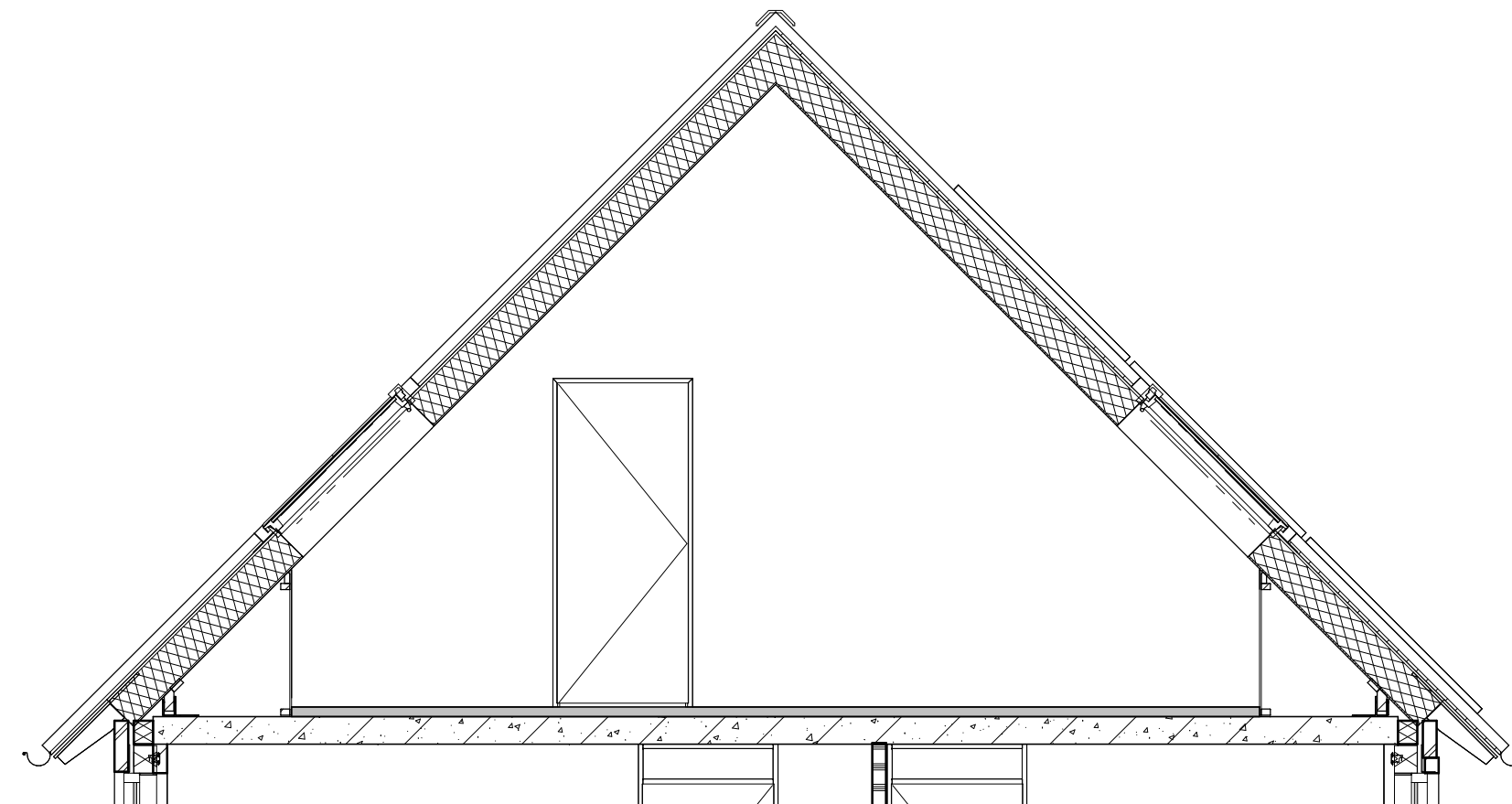
Doorsnede
