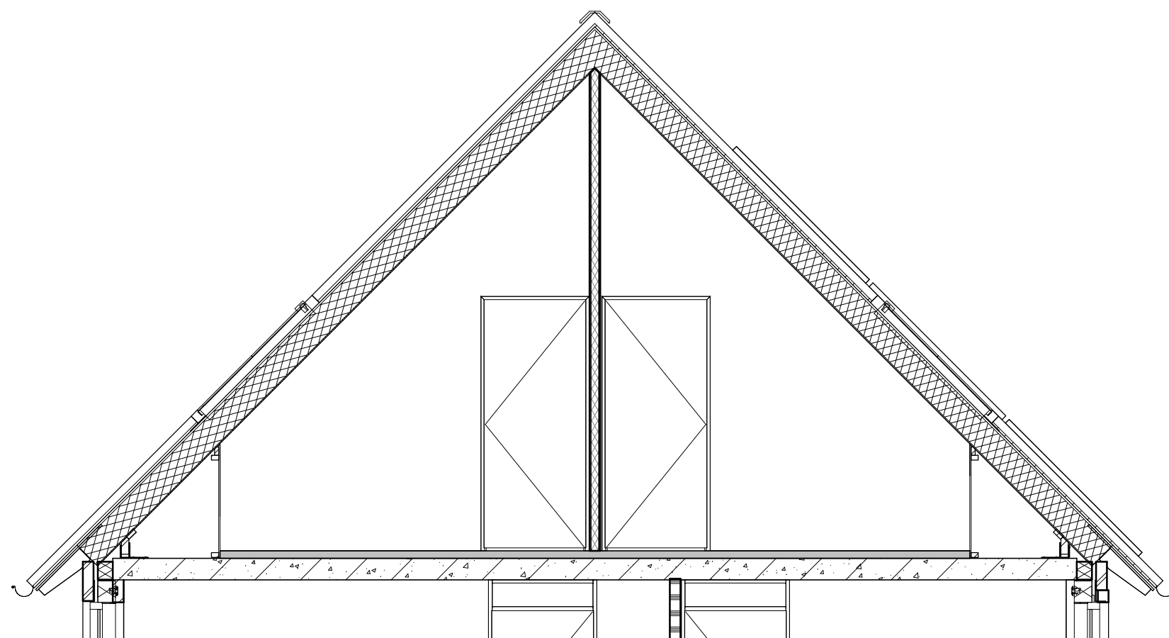
Doorsnede
