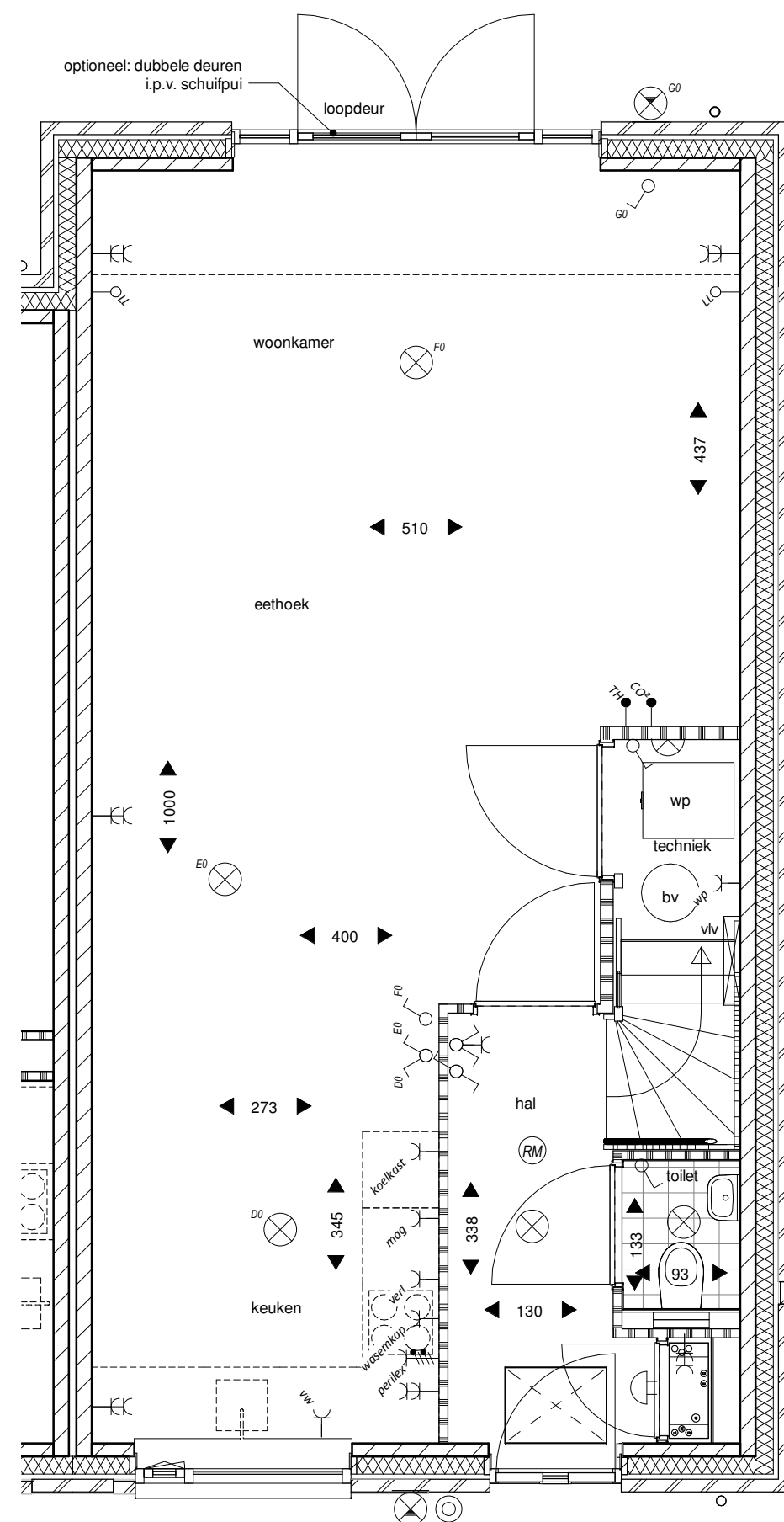
Begane grond
