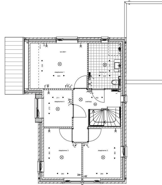
Eerste verdieping bouwnr 8
