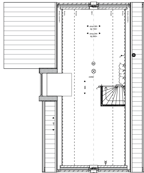
Tweede verdieping bouwnr 8
