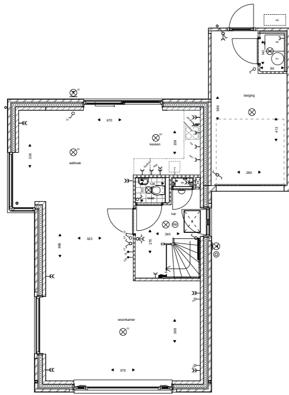
Begane grond bouwnr 8
