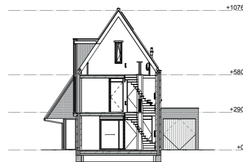
Doorsnede A
