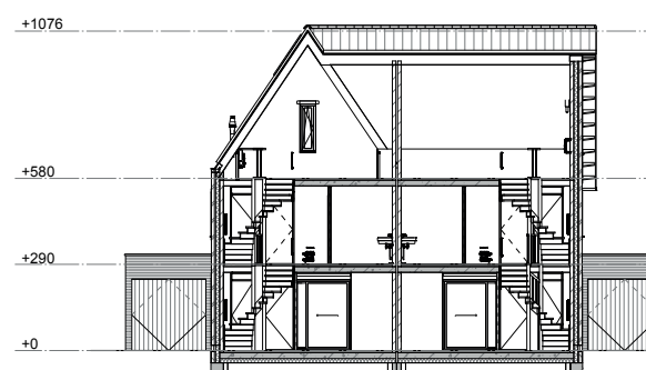
Doorsnede A
