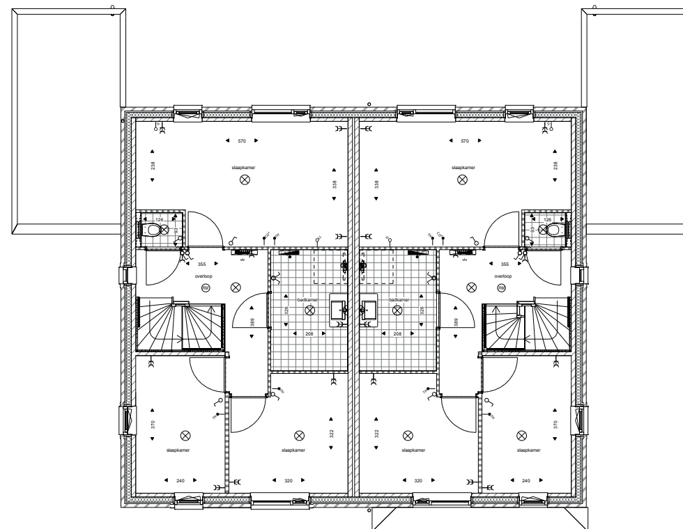
Eerste verdieping
