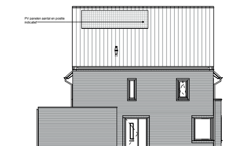
Linkergevel
