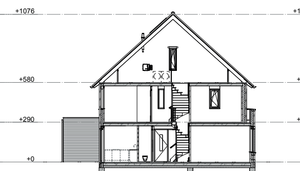
Doorsnede B
