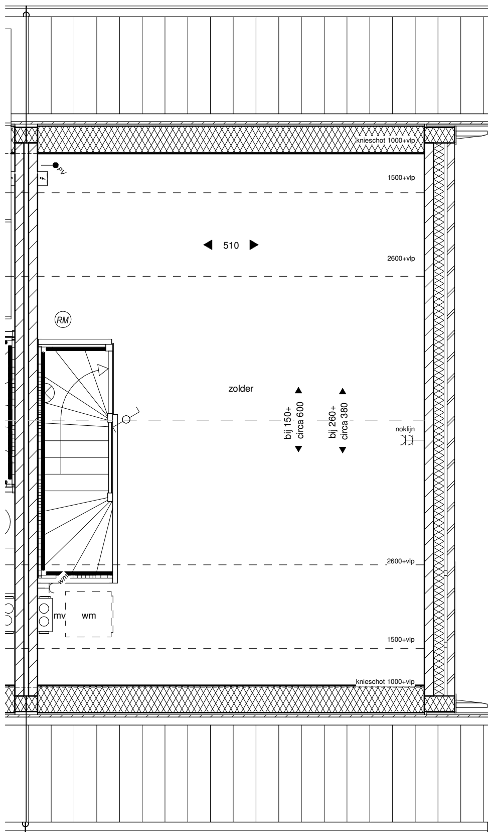
tweede verdieping
