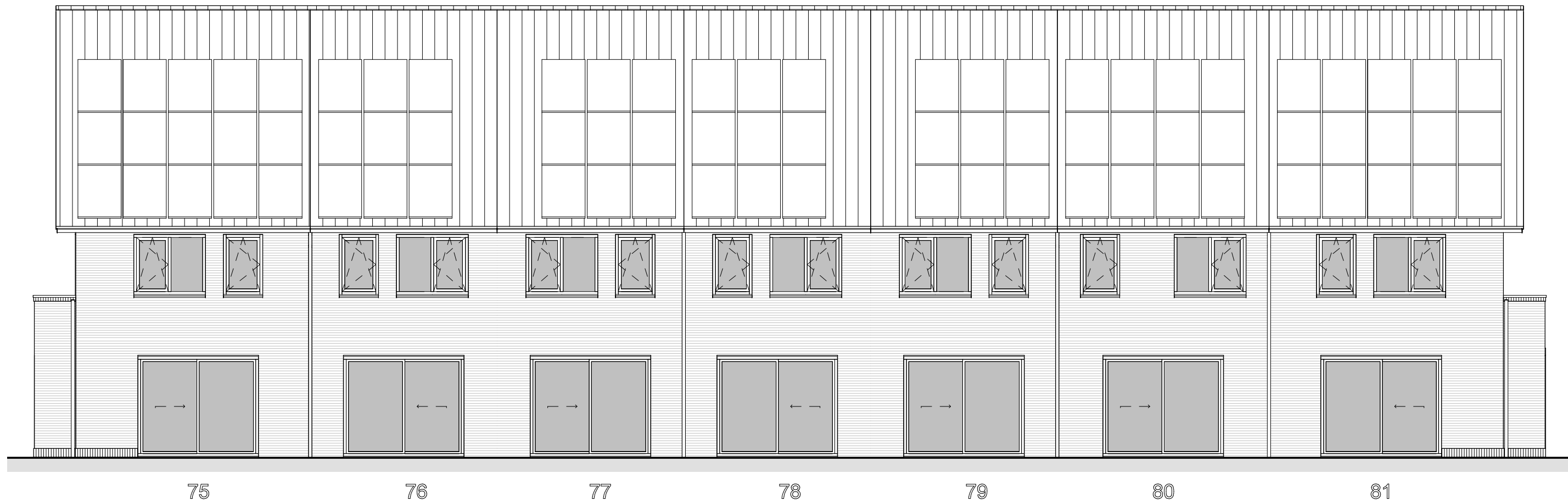
achtergevel
