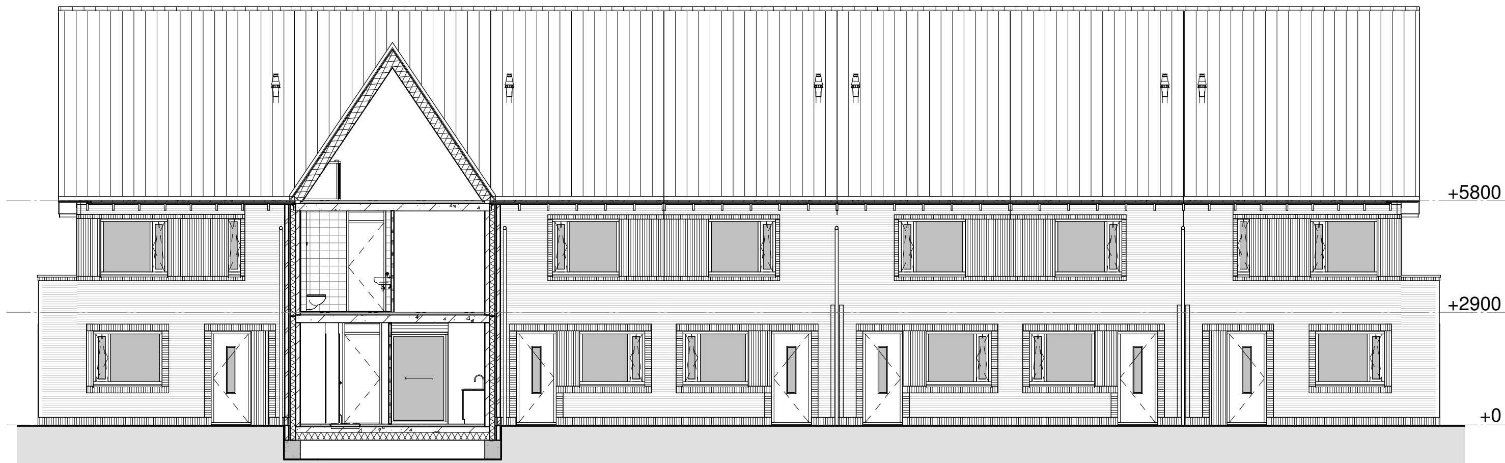
Doorsnede 16-B
