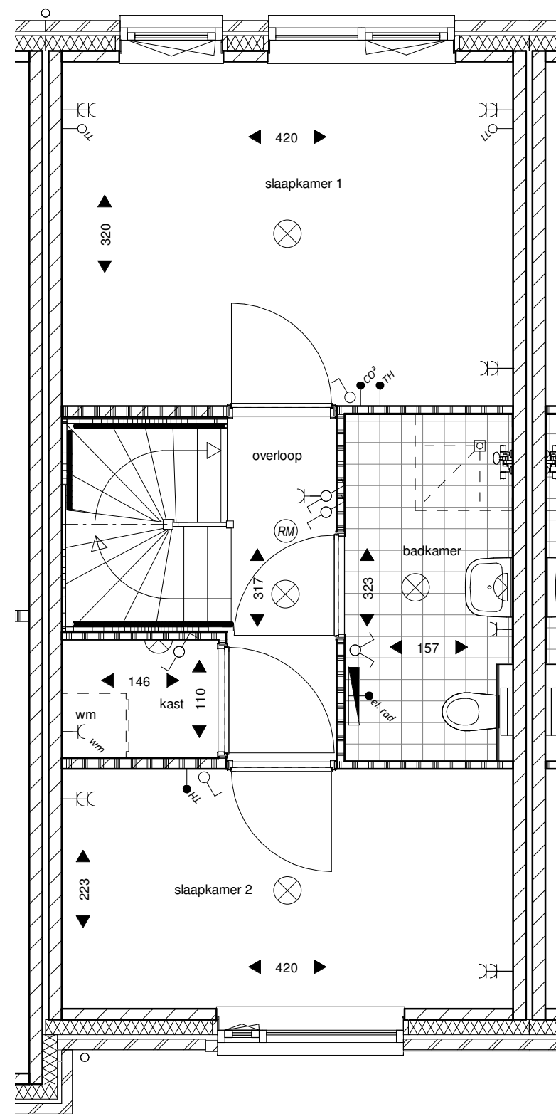
eerste verdieping
