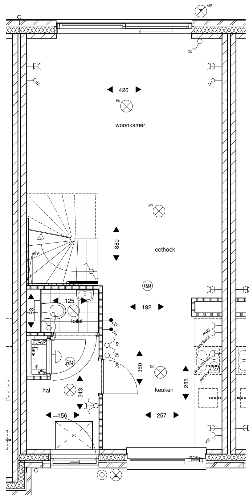
begane grond
