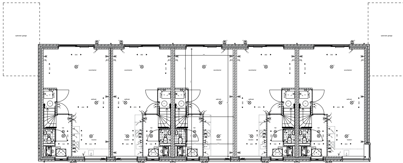
Begane grond bouwnr 47 bouwnr 46 bouwnr 45 bouwnr 44 bouwnr 43
