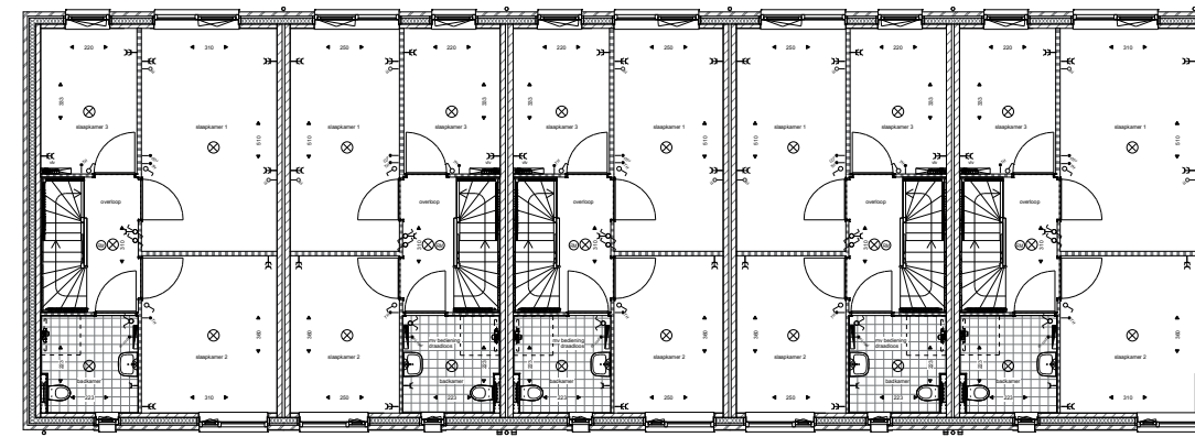
Eerste verdieping bouwnr 47 bouwnr 46 bouwnr 45 bouwnr 44 bouwnr 43
