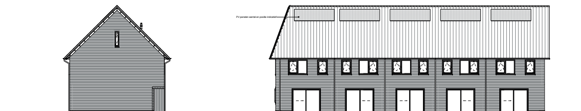
Linkergevel Achtergevel
