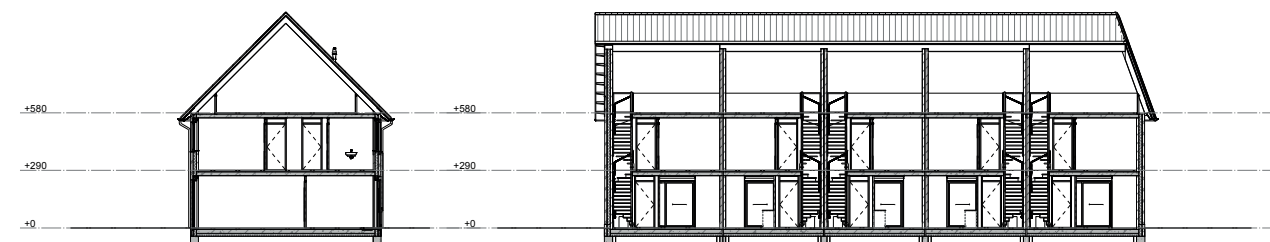
Doorsnede A Doorsnede B
