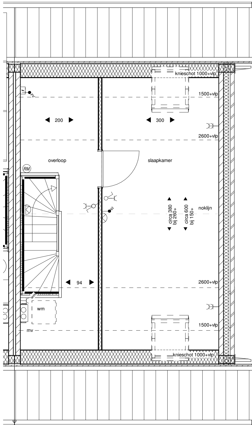
Tweede verdieping
