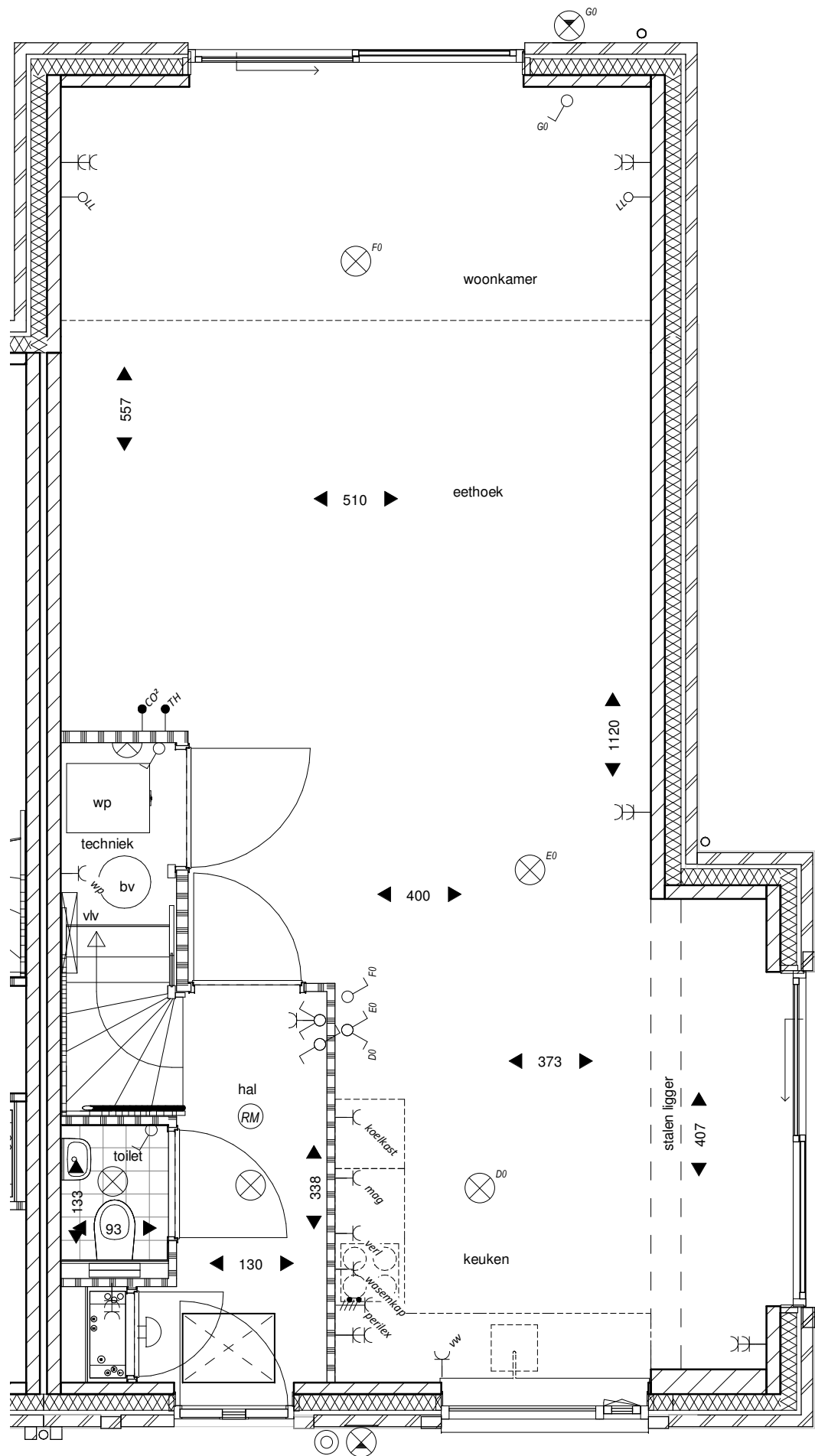
Begane grond
