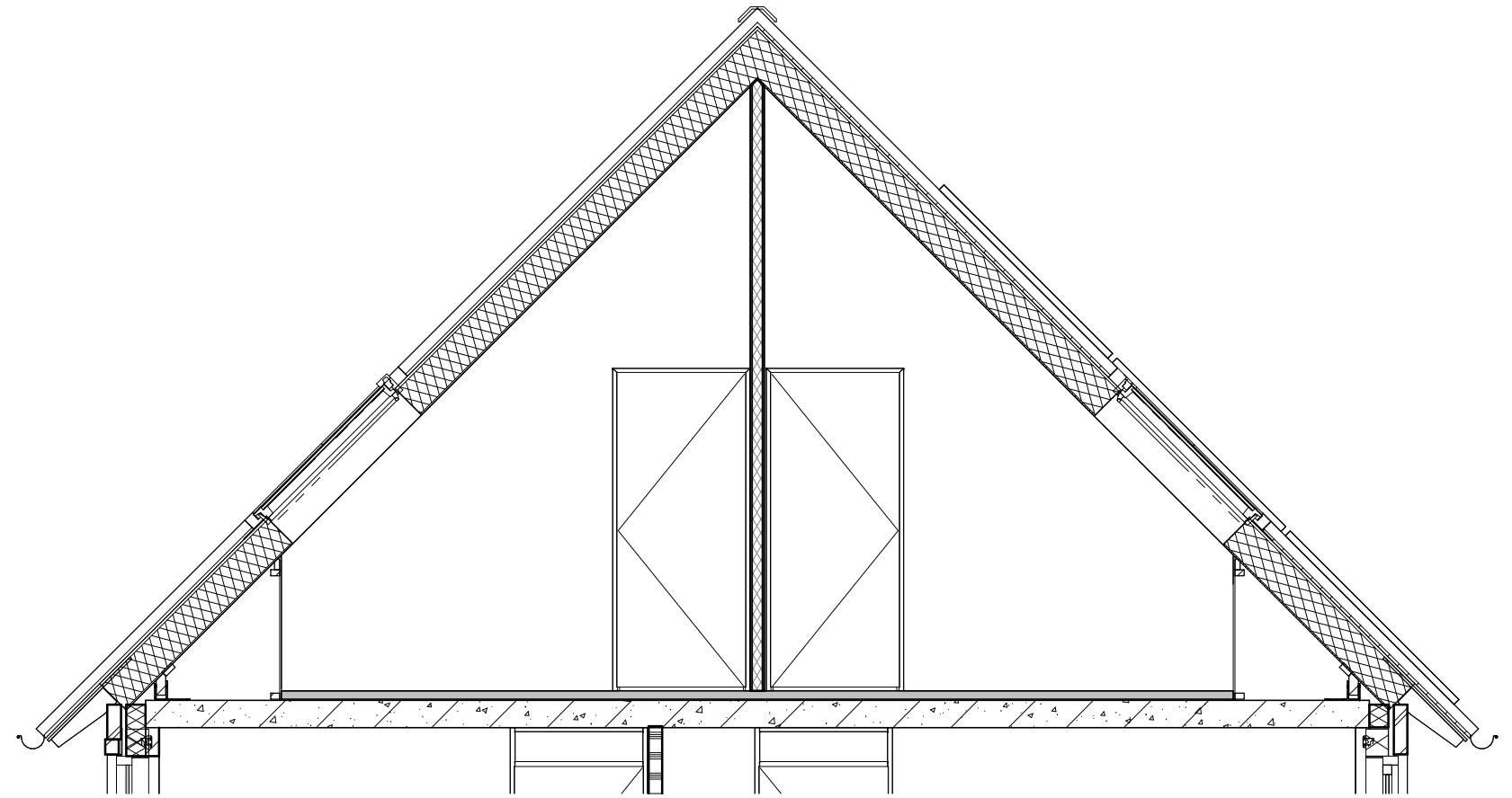
Doorsnede
