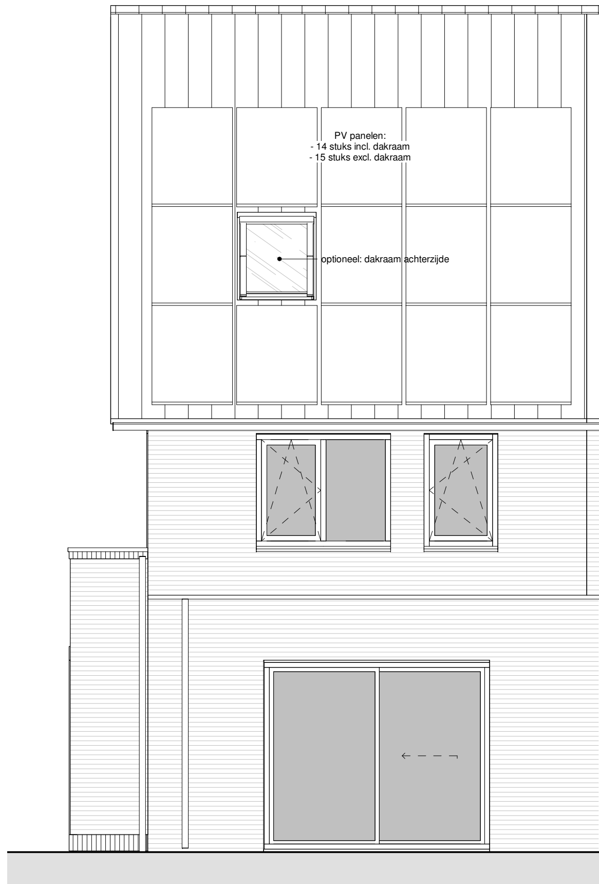
Achtergevel
