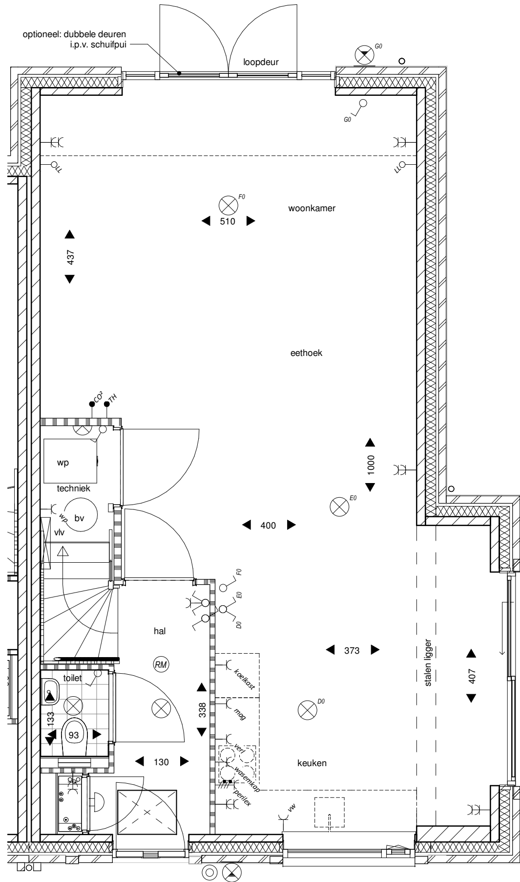
Begane grond
