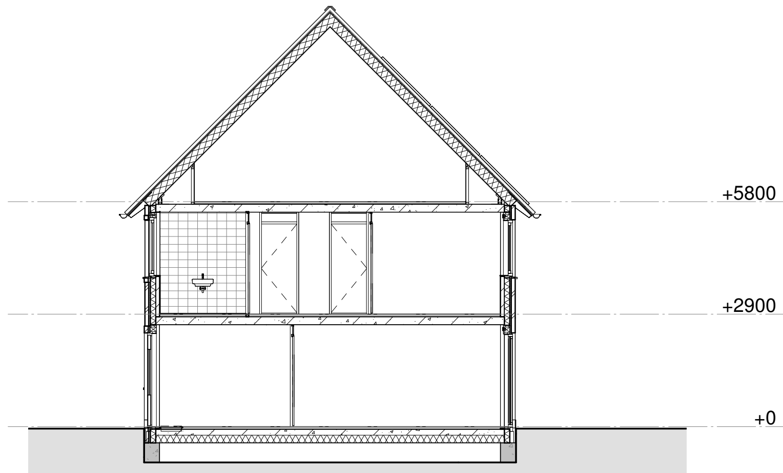
Doorsnede 14-A
