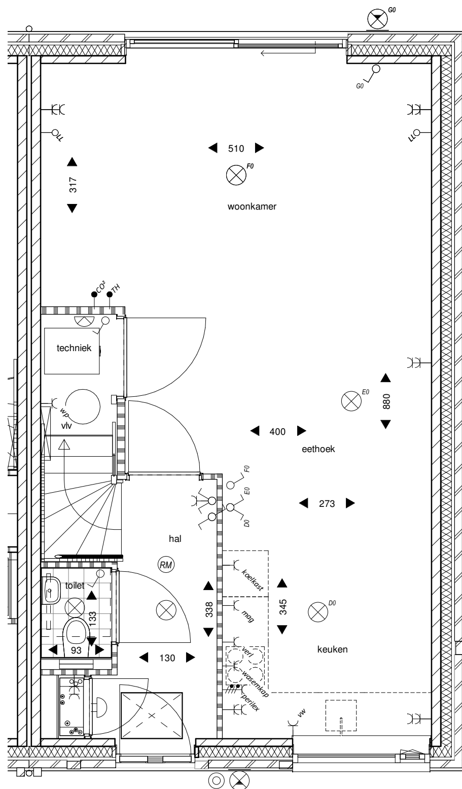
begane grond
