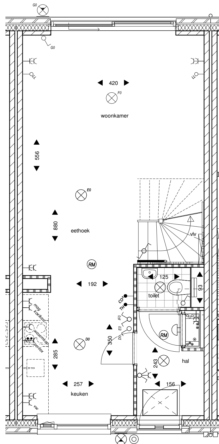
begane grond
