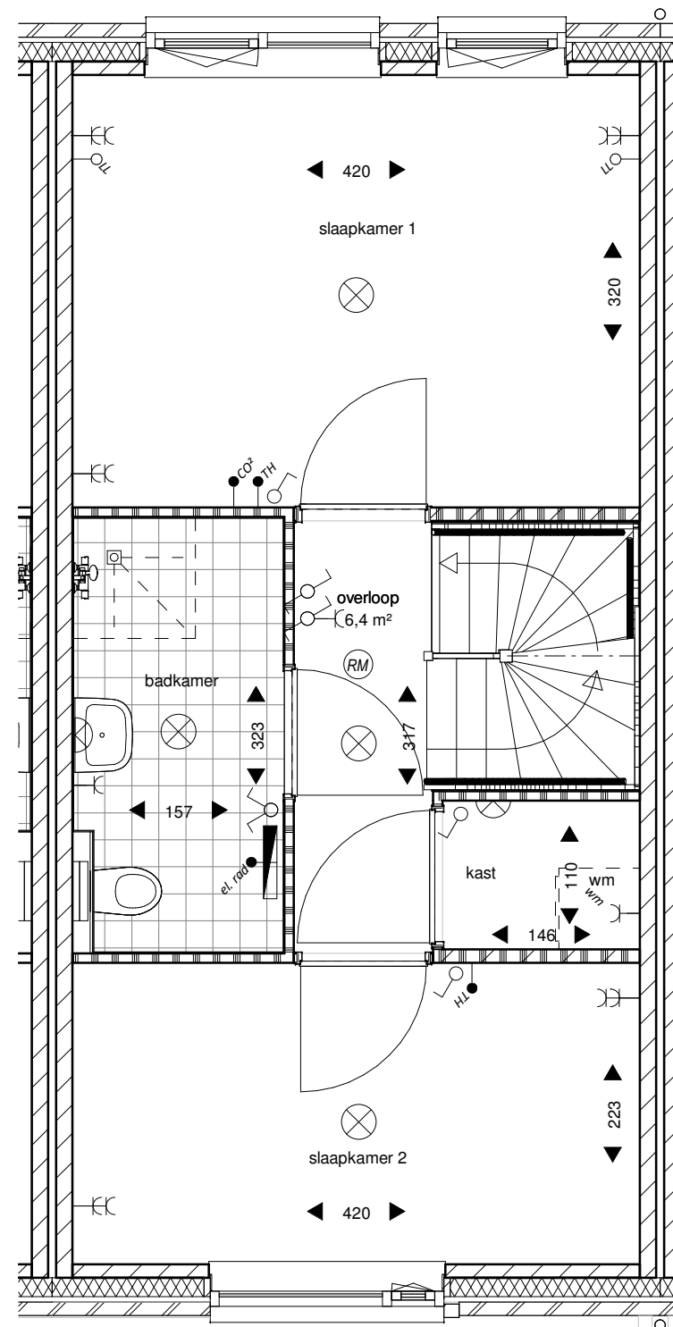
eerste verdieping
