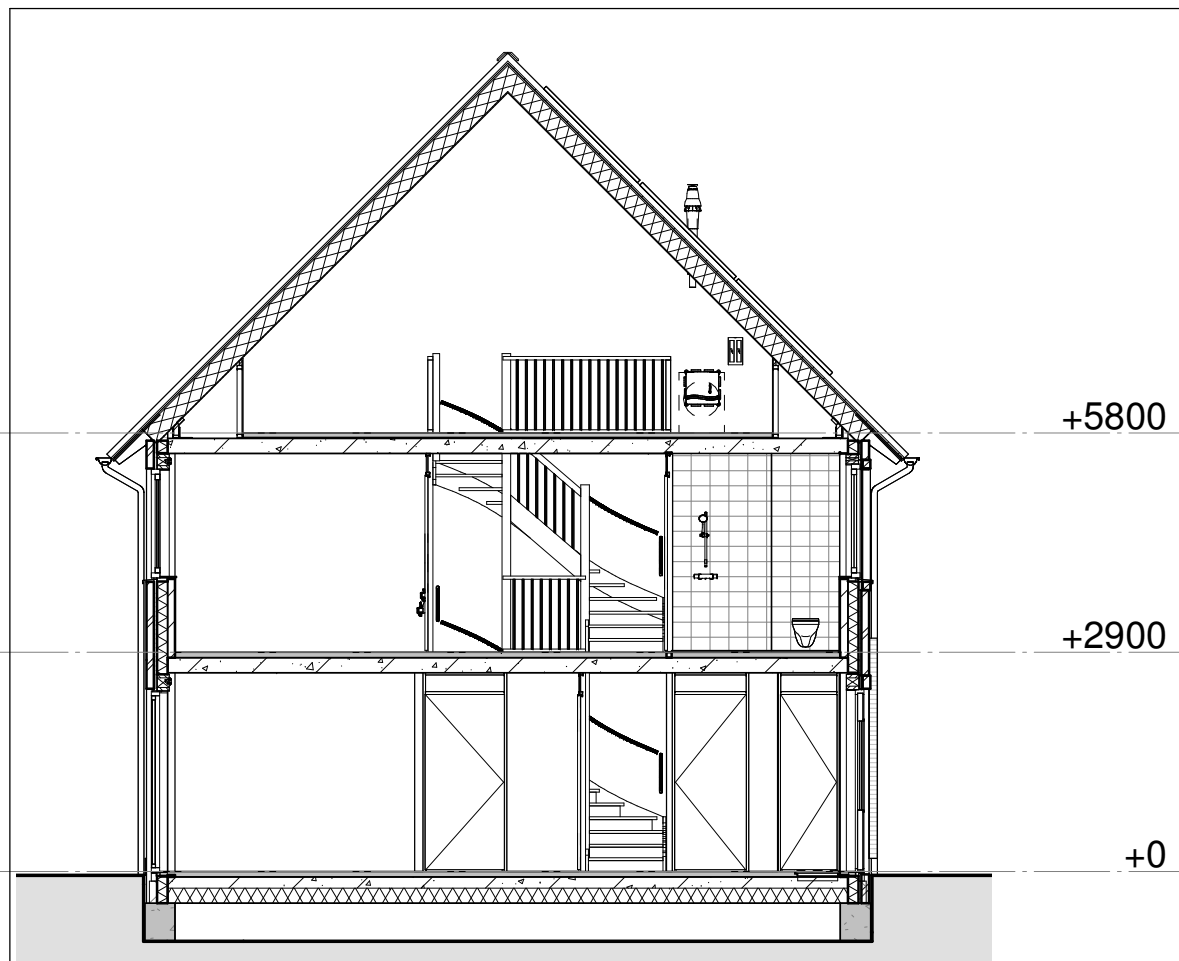
Doorsnede 19-A
