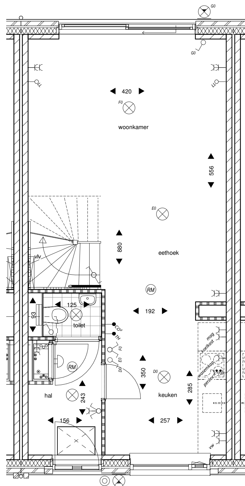
begane grond
