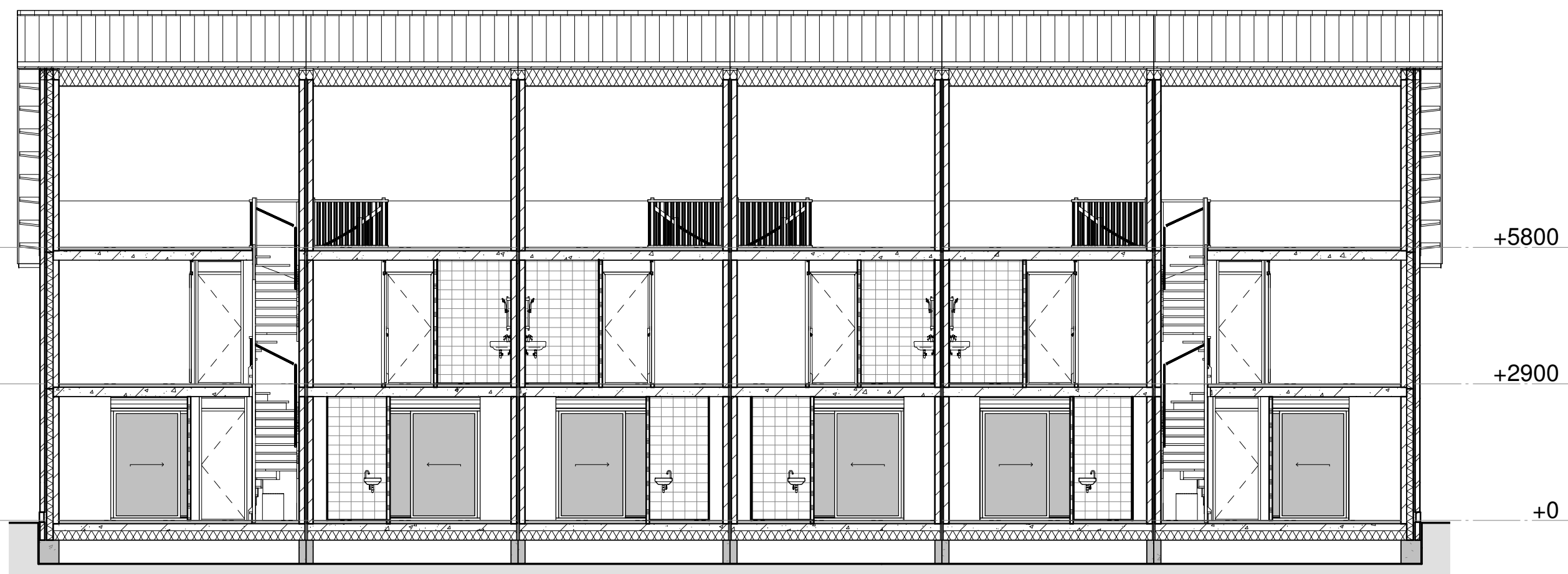
Doorsnede 19-B
