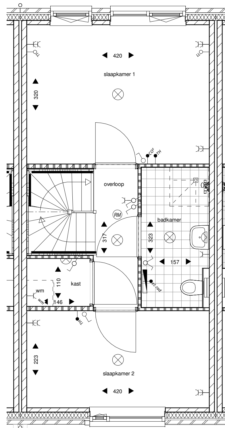
eerste verdieping
