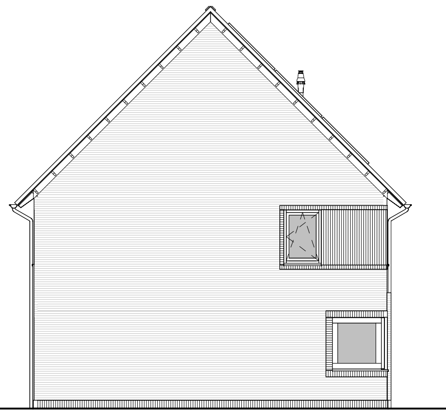
linkergevel
