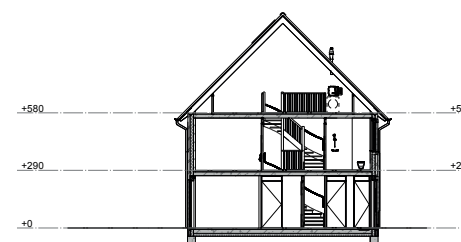
Doorsnede A
