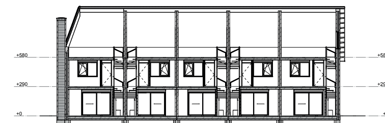
Doorsnede B
