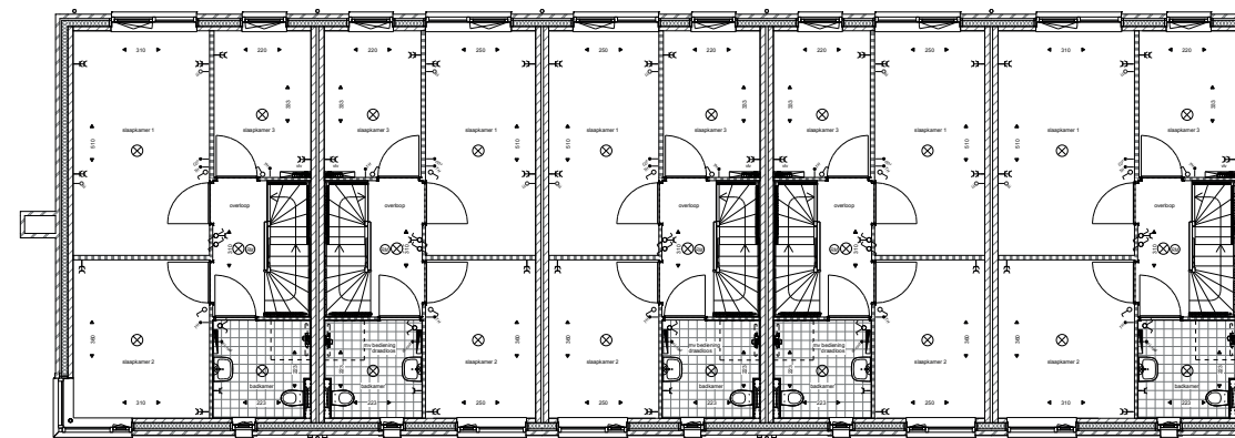
Eerste verdieping
